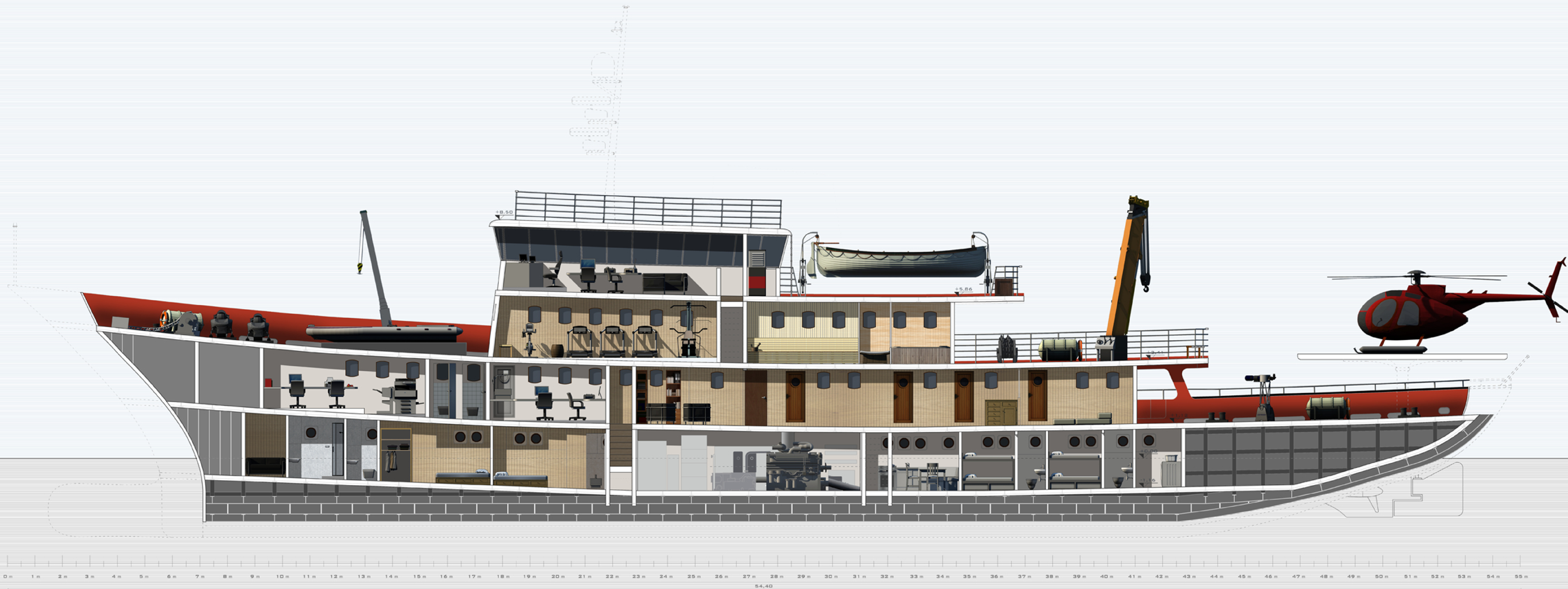
SEZIONE B-B SCALA 1:50
