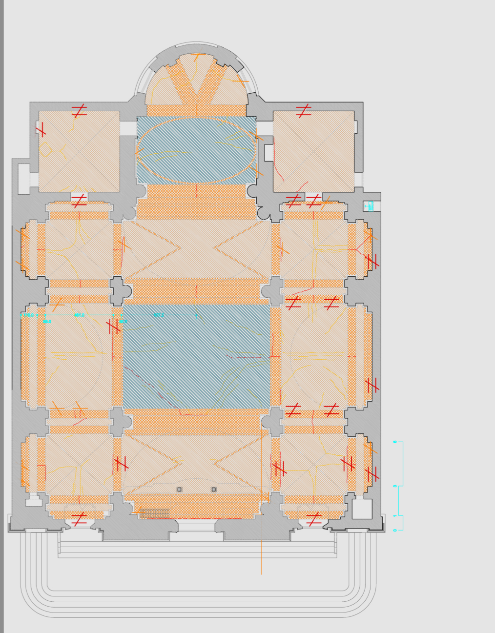
PIANTA DELLE LESIONI ALLE VOLTE
