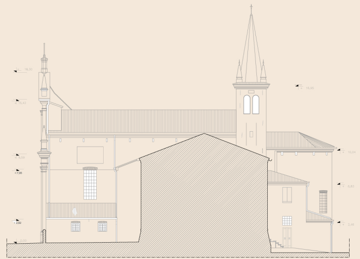
PROSPETTO EST
