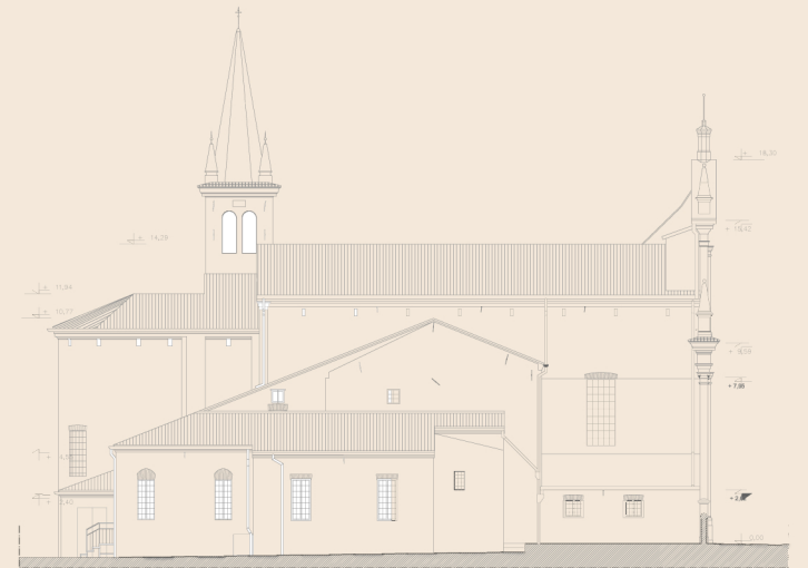
PROSPETTO OVEST
