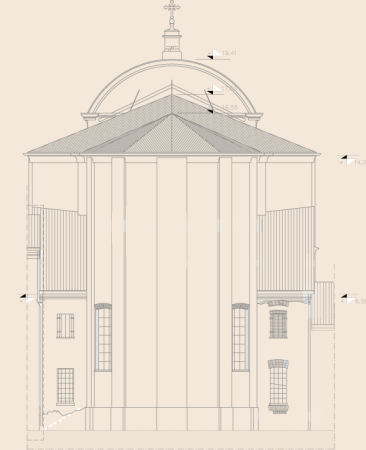
PROSPETTO EST
