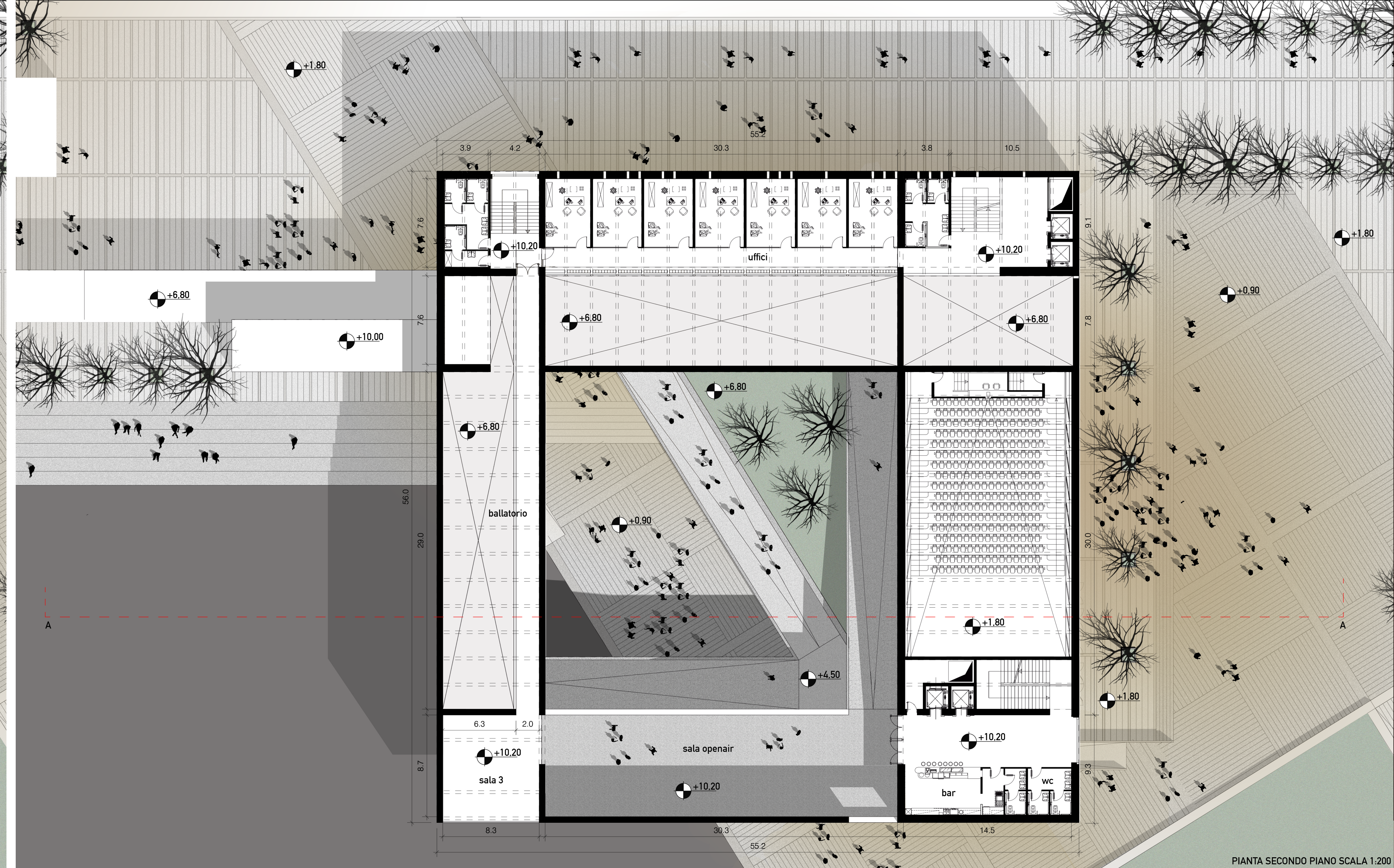
PIANTA SECONDO PIANO SCALA 1:200
