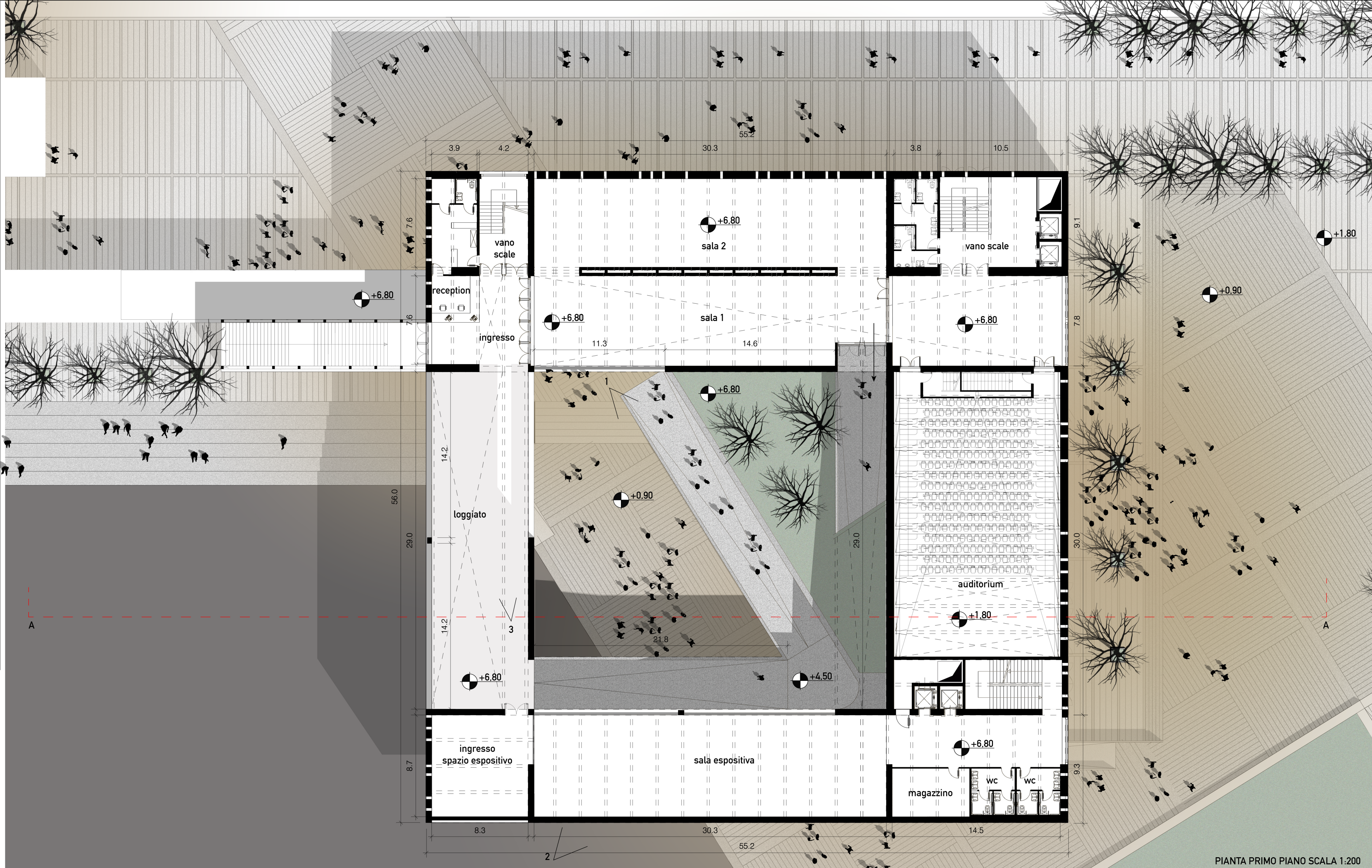
PIANTA PRIMO PIANO SCALA 1:200
