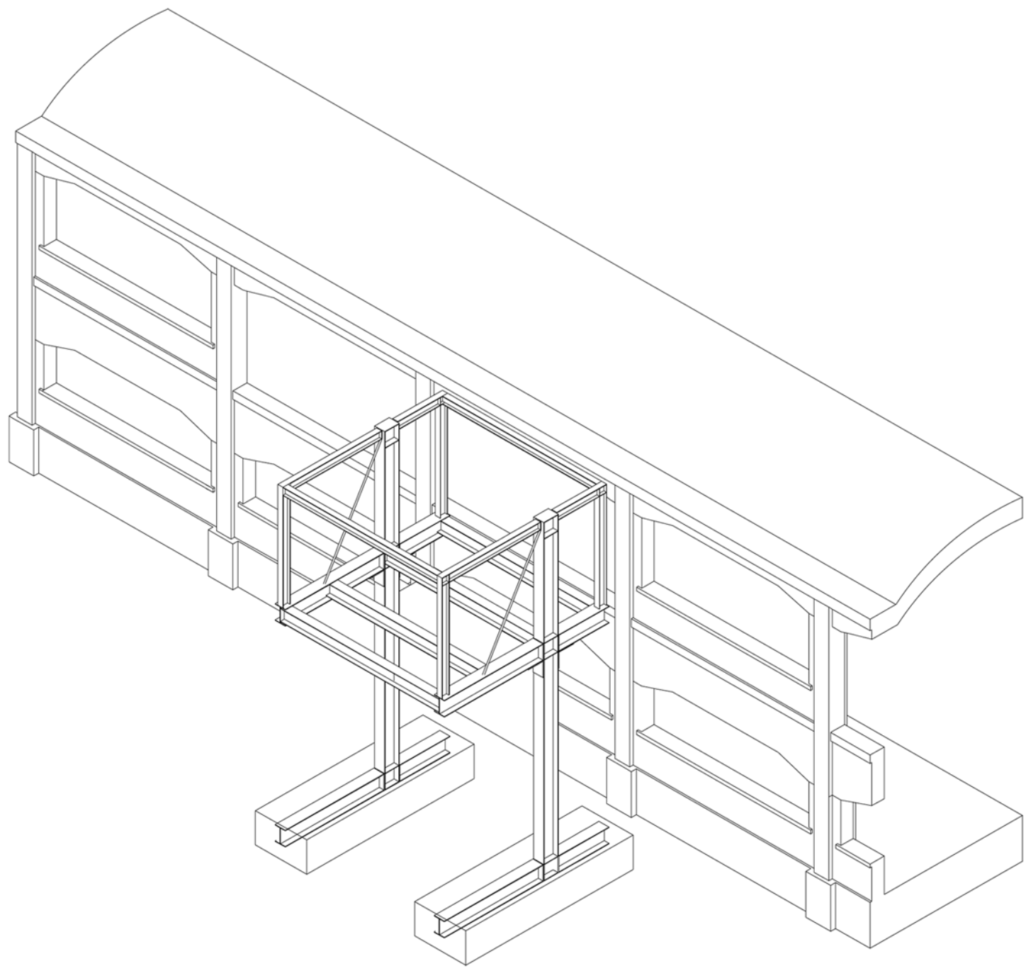
GABBIA STRUTTURALE CON PROFILI IN ACCIAIO
