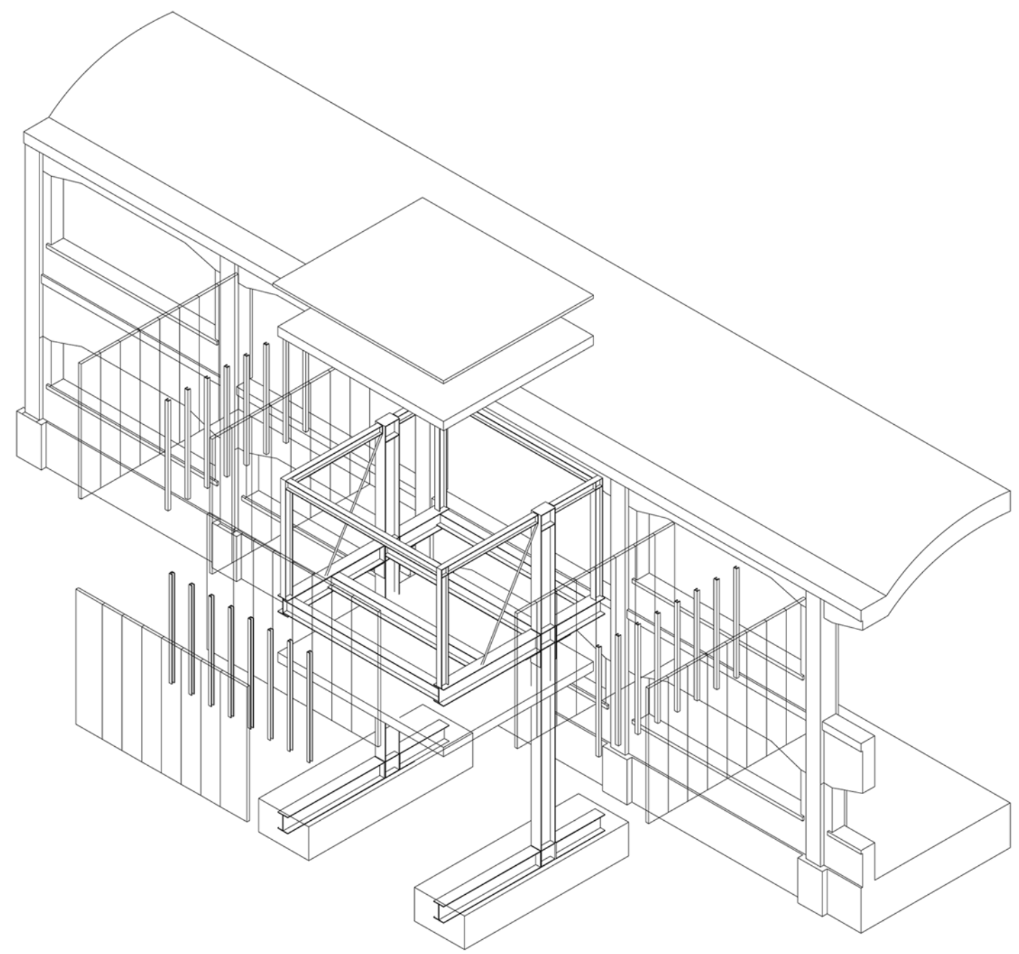
MONTAGGIO PACCHETTO CHIUSURE VERTICALI policarbonato_telaio con intercapedine d'aria_policarbonato
