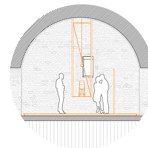
Esempio sala 1:100
