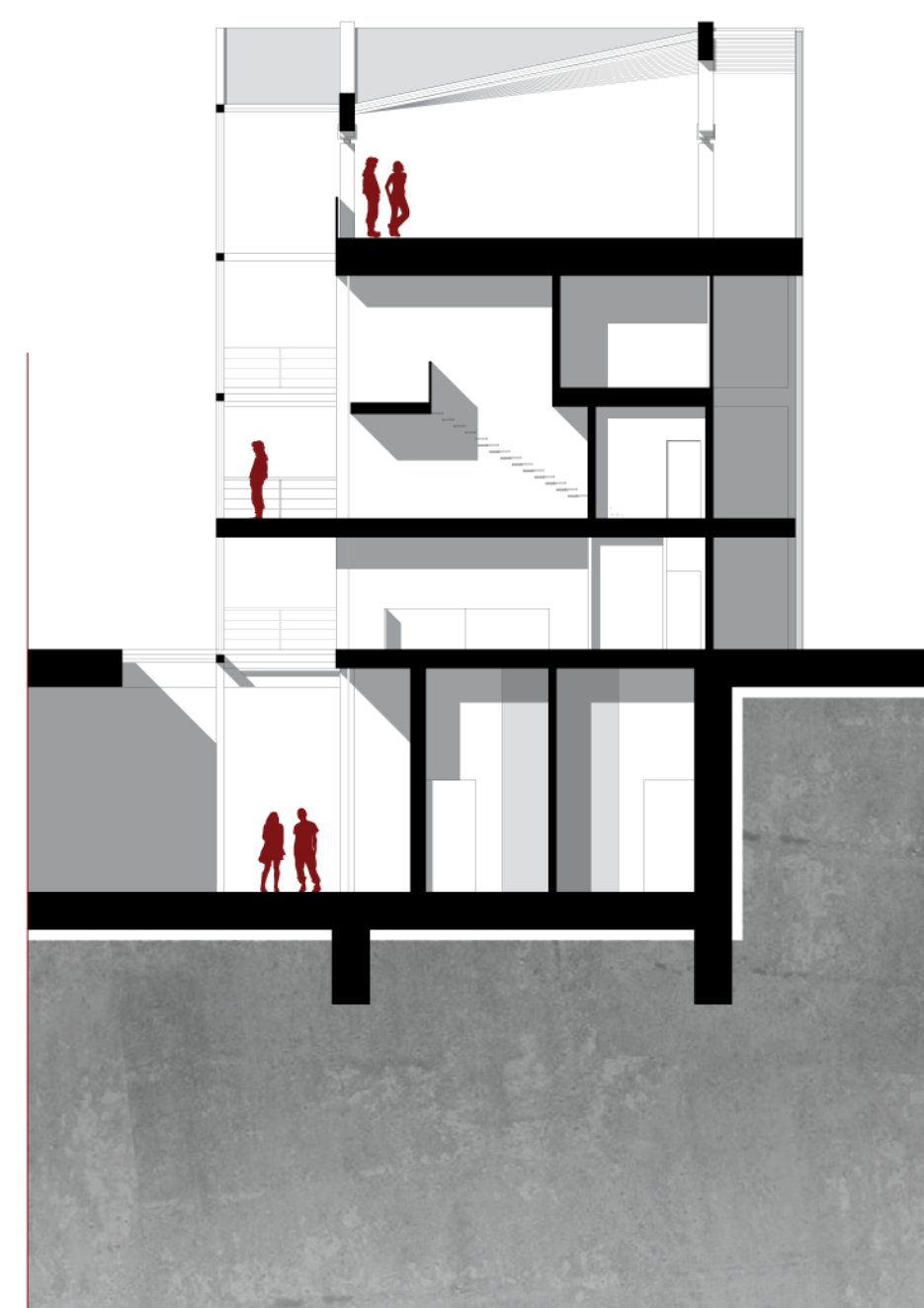
SEZIONE TRASVERSALE C-C'
