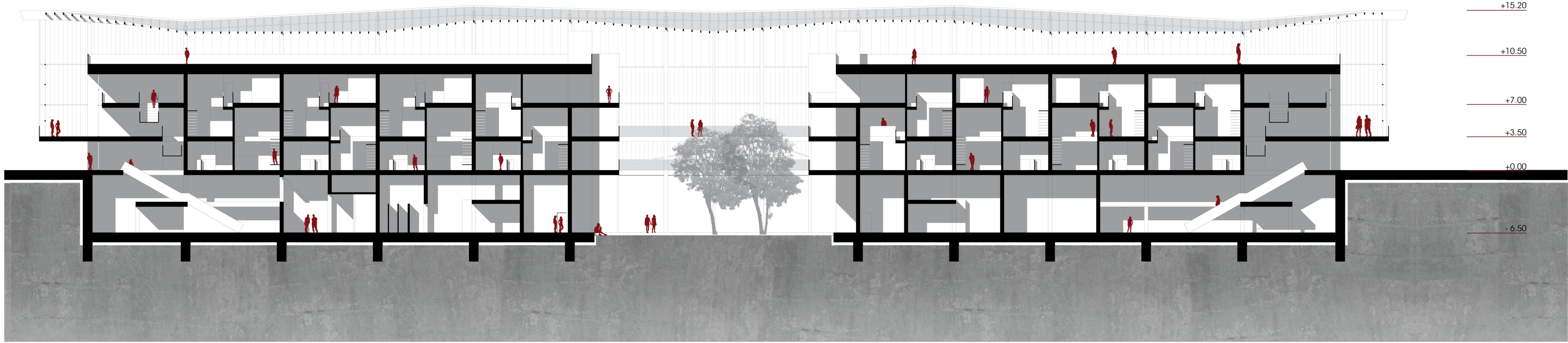
SEZIONE LONGITUDINALE A-A'
