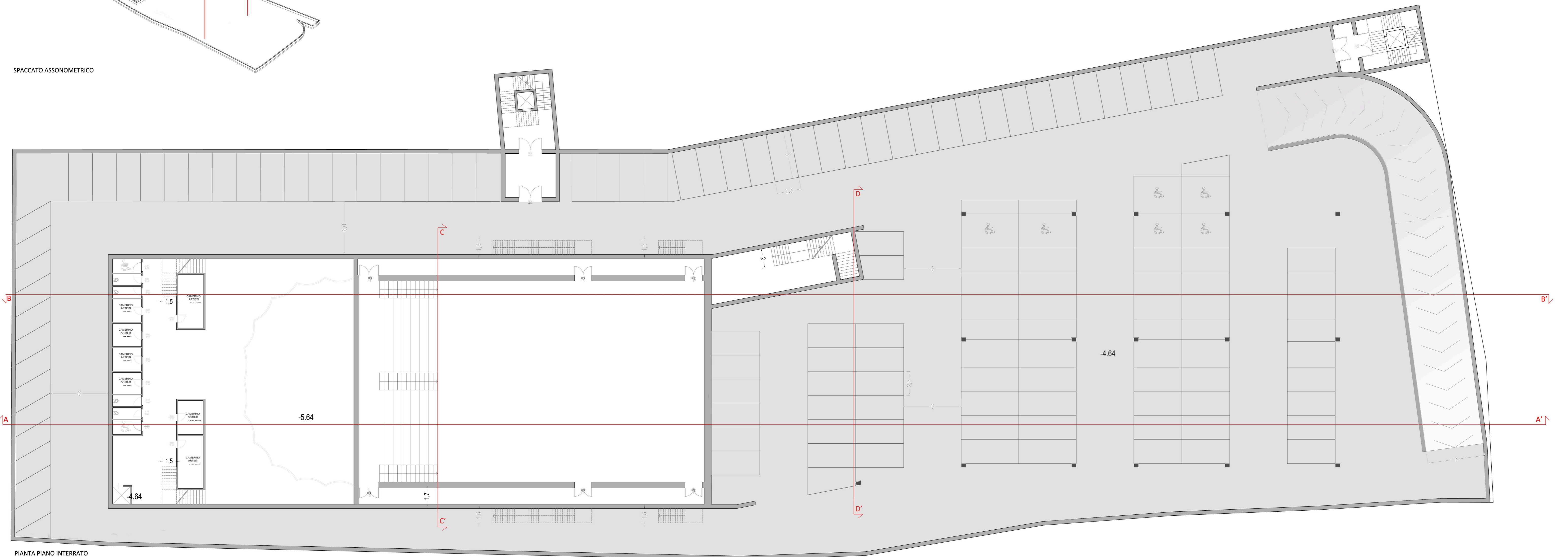
PIANTA PIANO INTERRATO
