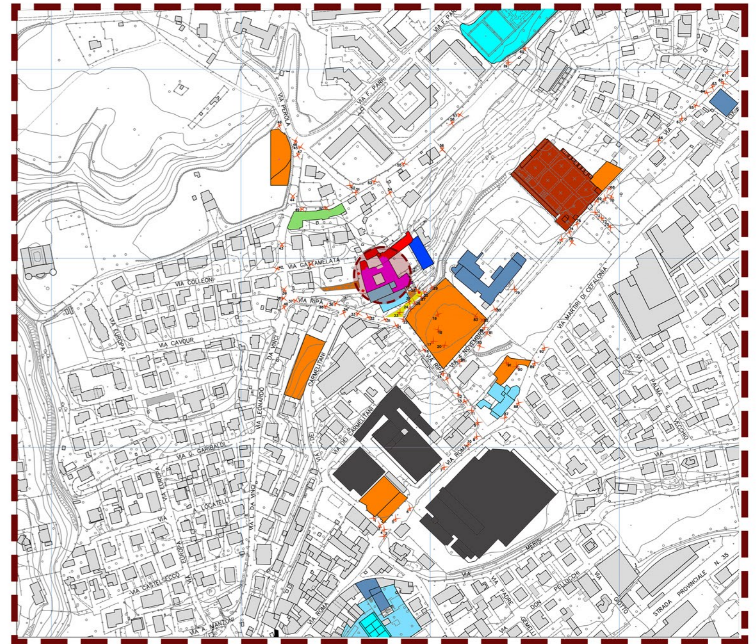
INQUADRAMENTO EX MONASTERO DELLA RIPA SCALA 1:500
