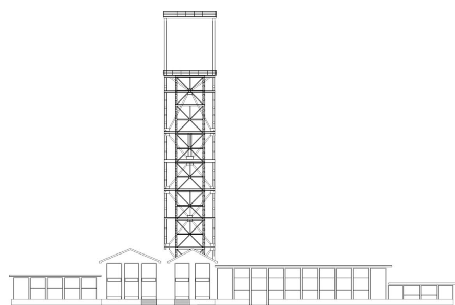
partido estructural primario
