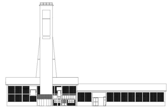
elevación norte galpon sur
