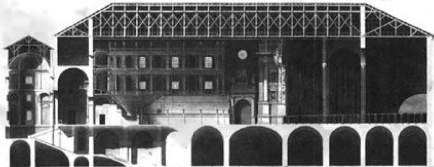
Coupe sur la hauteur du grand Theatre de Parme ALEOTTI
