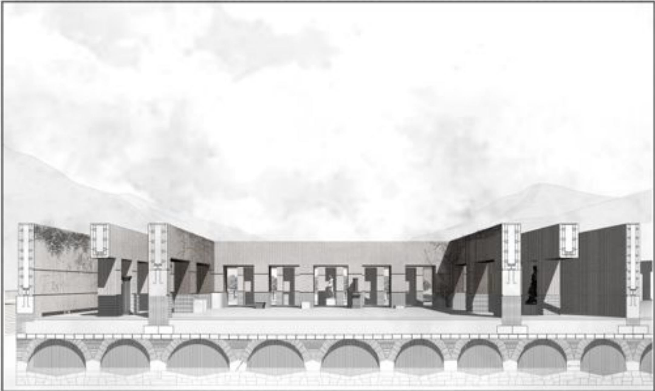
SEZIONE PROSPETTICA DELLE PALESTRE O ISEUM
