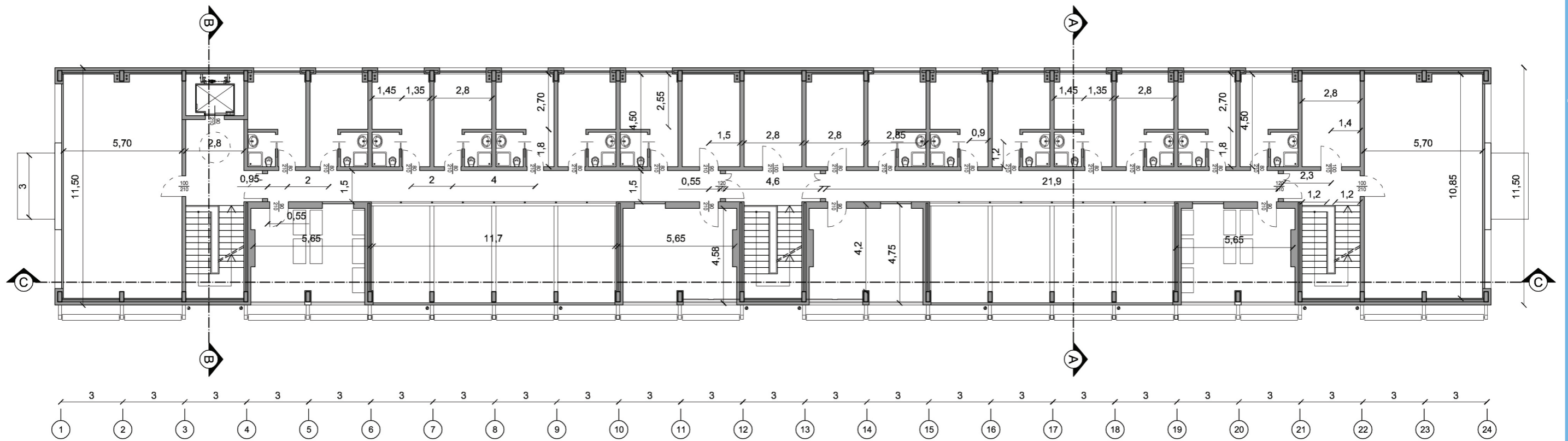
PIANO PRIMO
