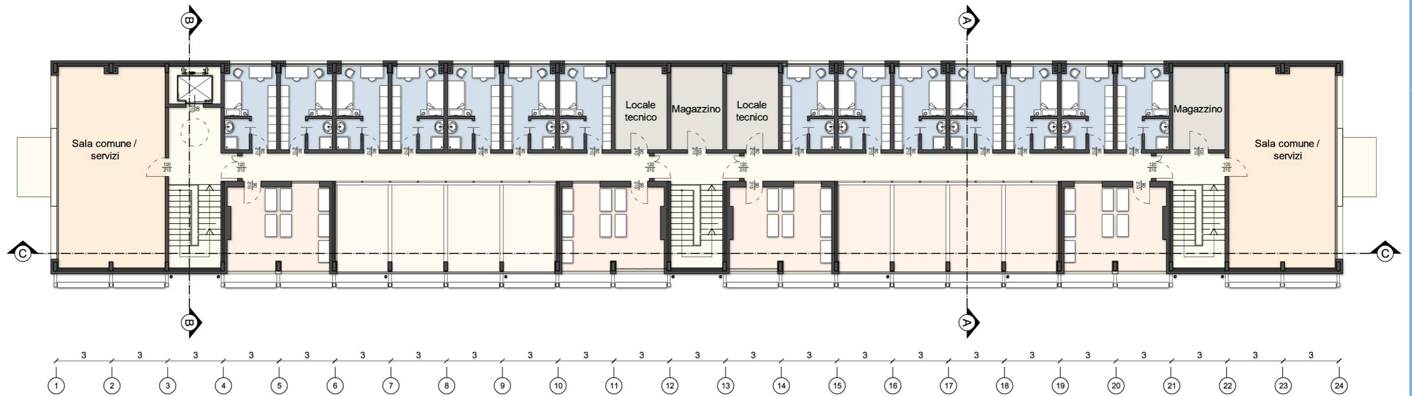
PIANO PRIMO
