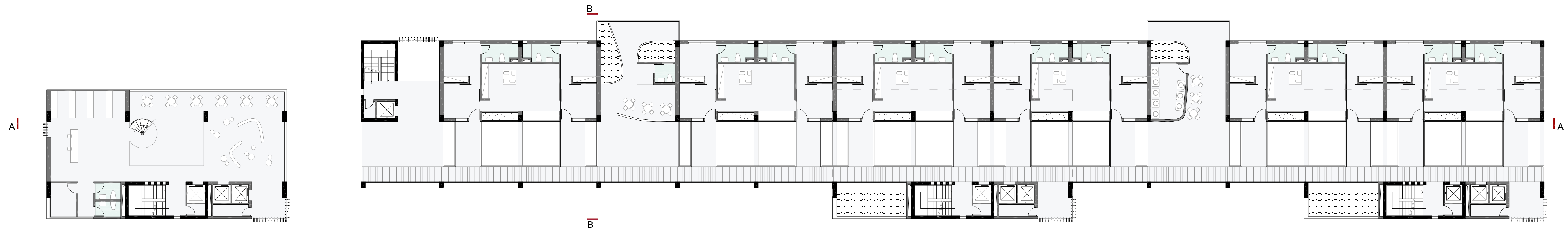
Pianta quota +14,40 Cohousing e livello inferiore della biblioteca di quartiere
