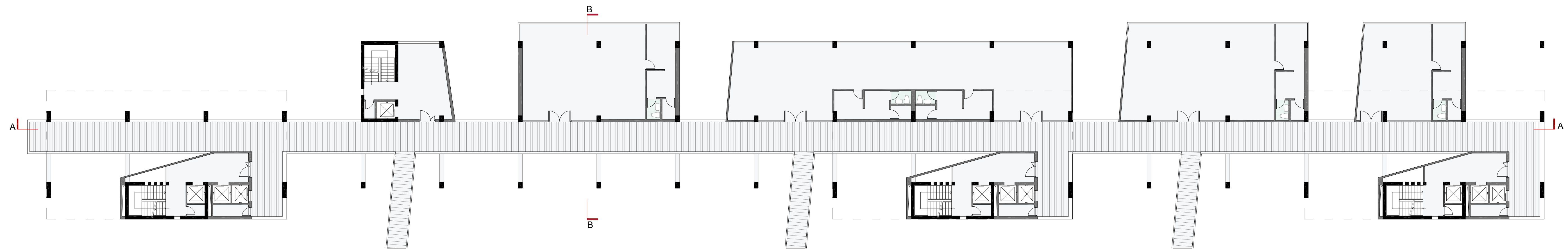
Pianta quota +14,40 Cohousing e livello inferiore della biblioteca di quartiere
