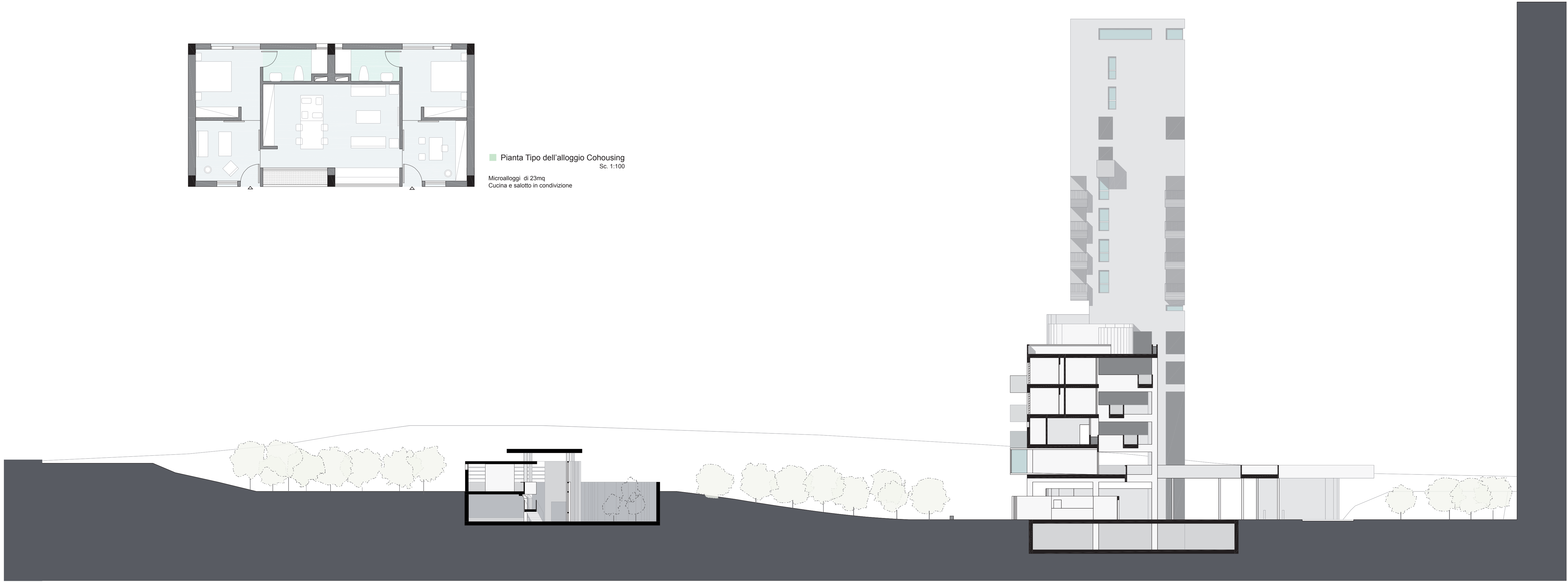
Sezione Trasversale BB' Sc. 1:200
