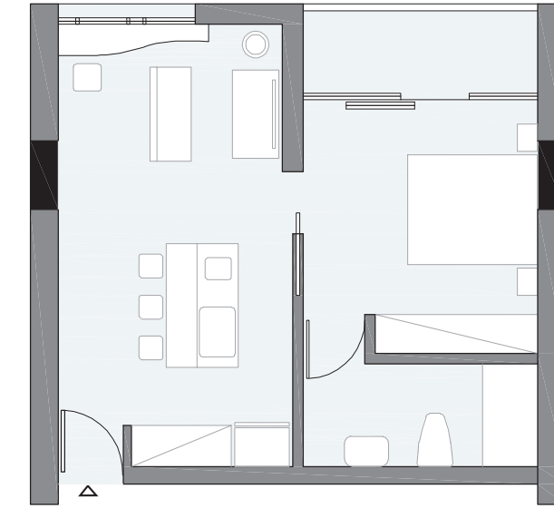
Bilocale (43mq) Sc. 1:100
