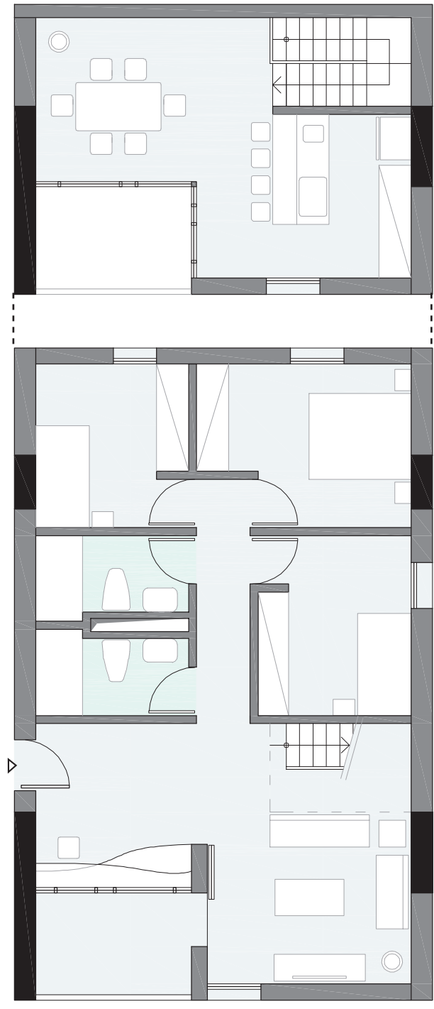
Duplex Tipo B (103mq) Sc. 1:100
