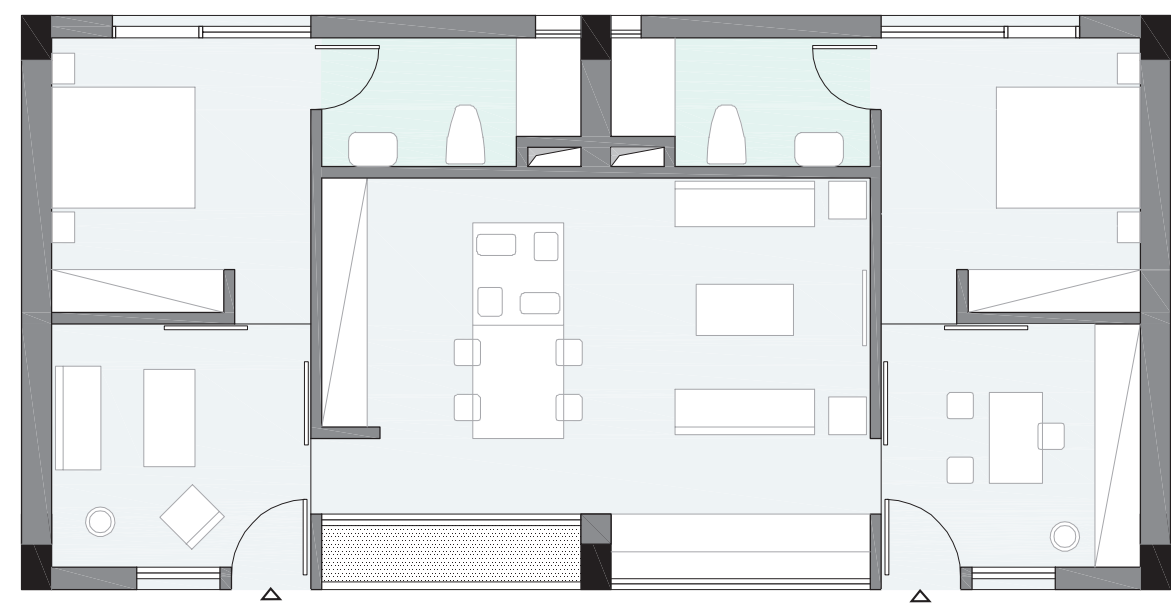
Pianta Tipo dell'alloggio Cohousing Sc. 1:100
