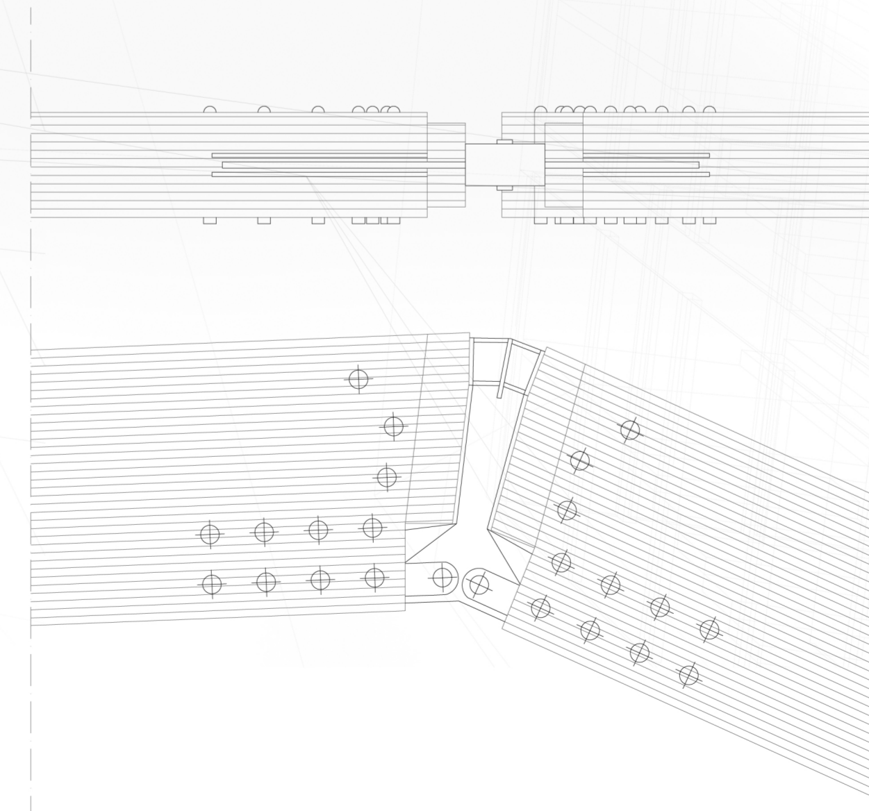
DETTAGLIO NODO RIGIDO TRAVI DI COPERTURA CENTRALI 1:20
