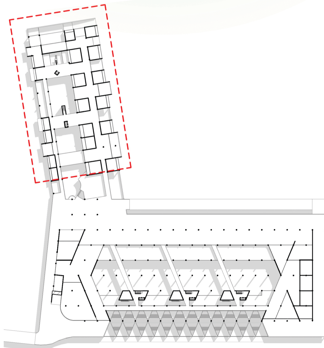
Primo Piano Livello +3.84
