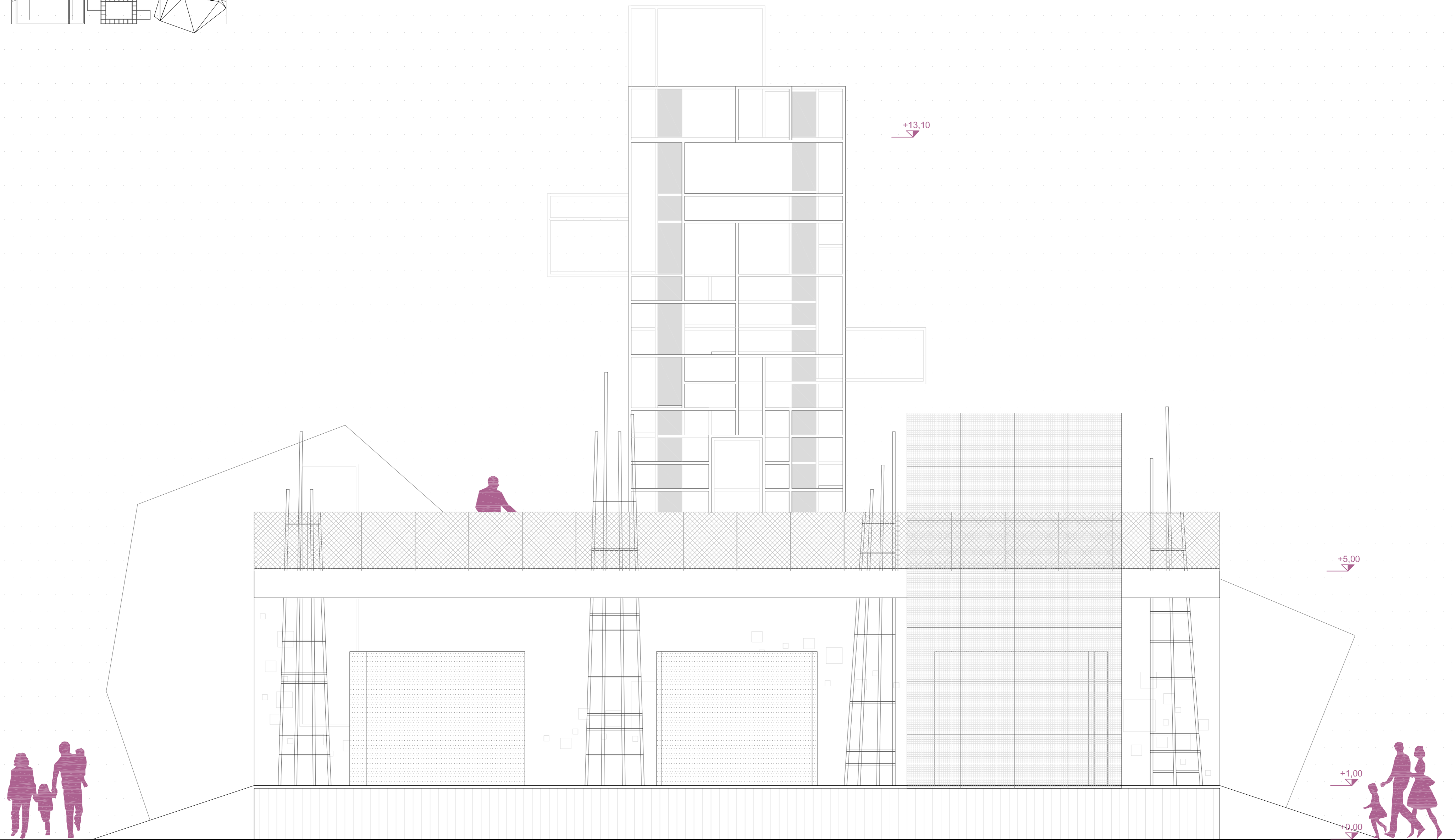
PROSPETTO 02 - scala 1-50
