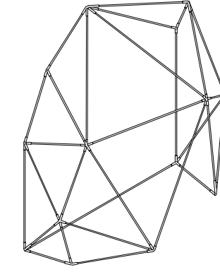
telo interno tubolari in acciaio cavi Ø5cm
