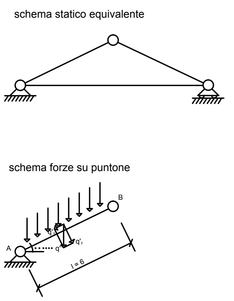
COPERTURA ESISTENTE
