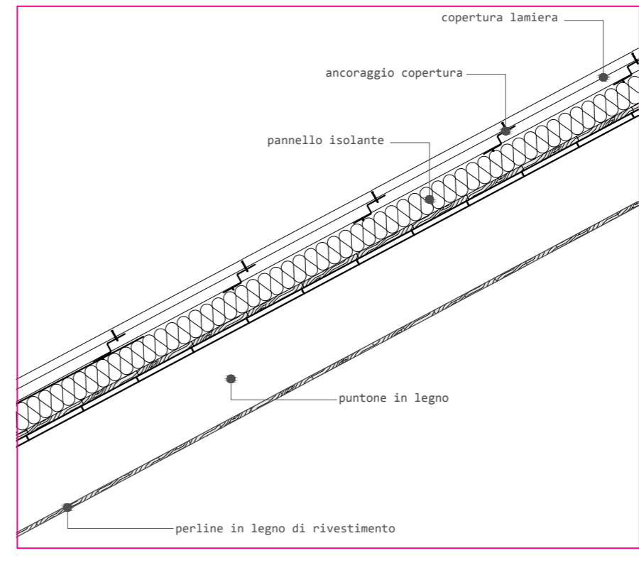
COPERTURA PROGETTO
