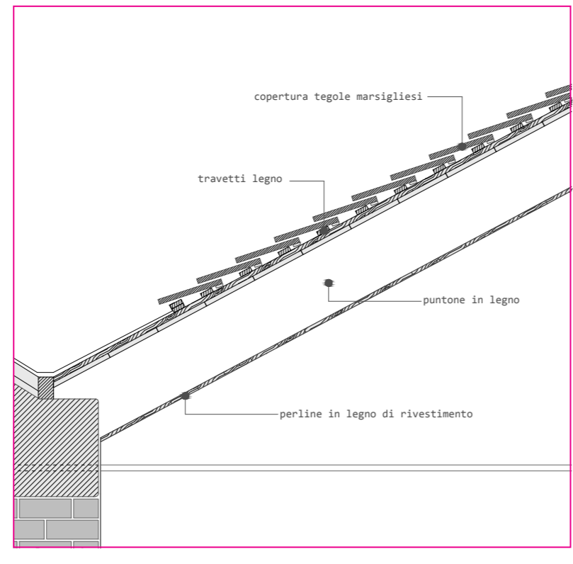
COPERTURA ESISTENTE
