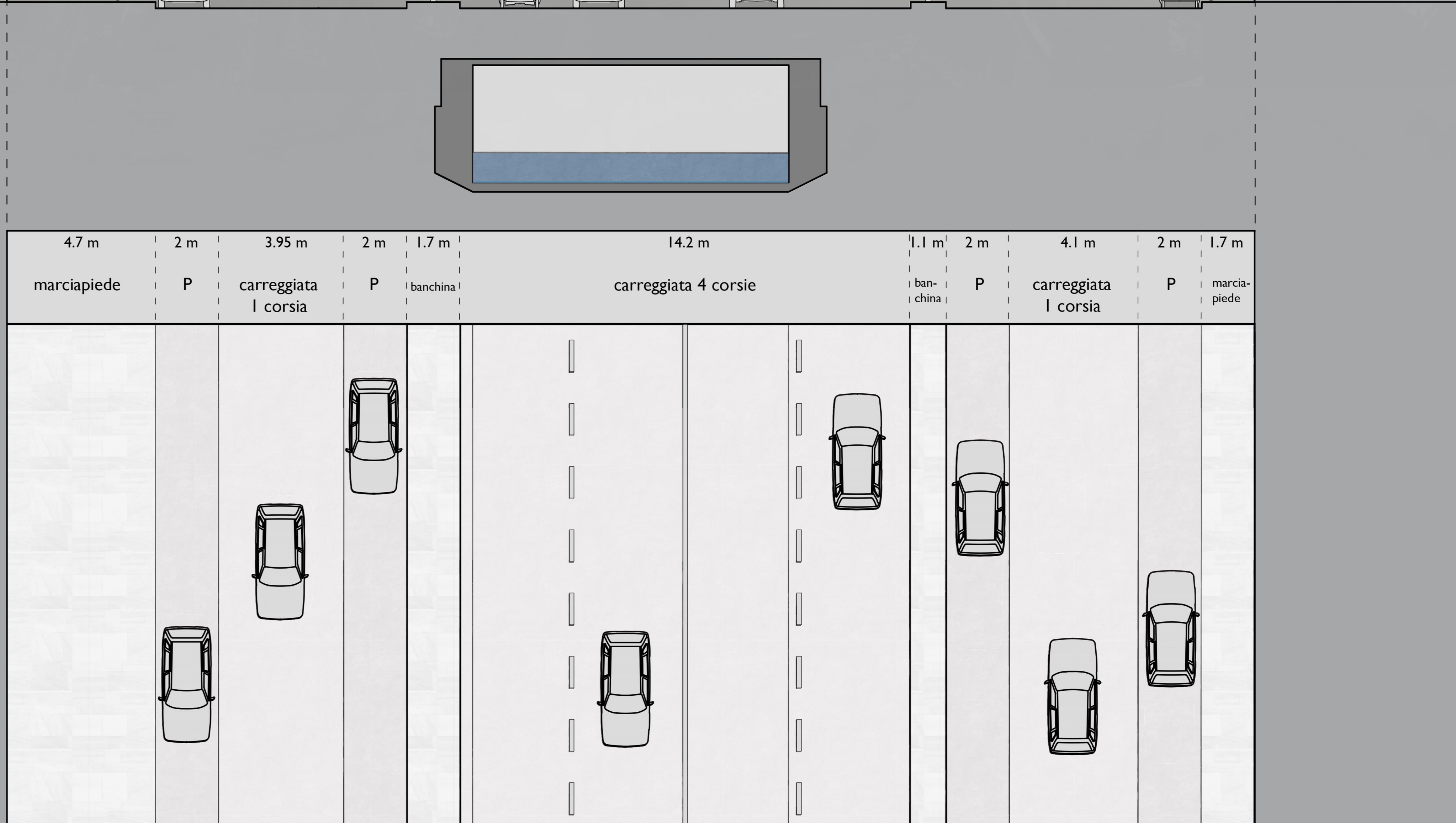
In ordine dall'alto verso il basso: - Ortofoto dell'area di progetto - Sezione e pianta stradali della stato di fatto
