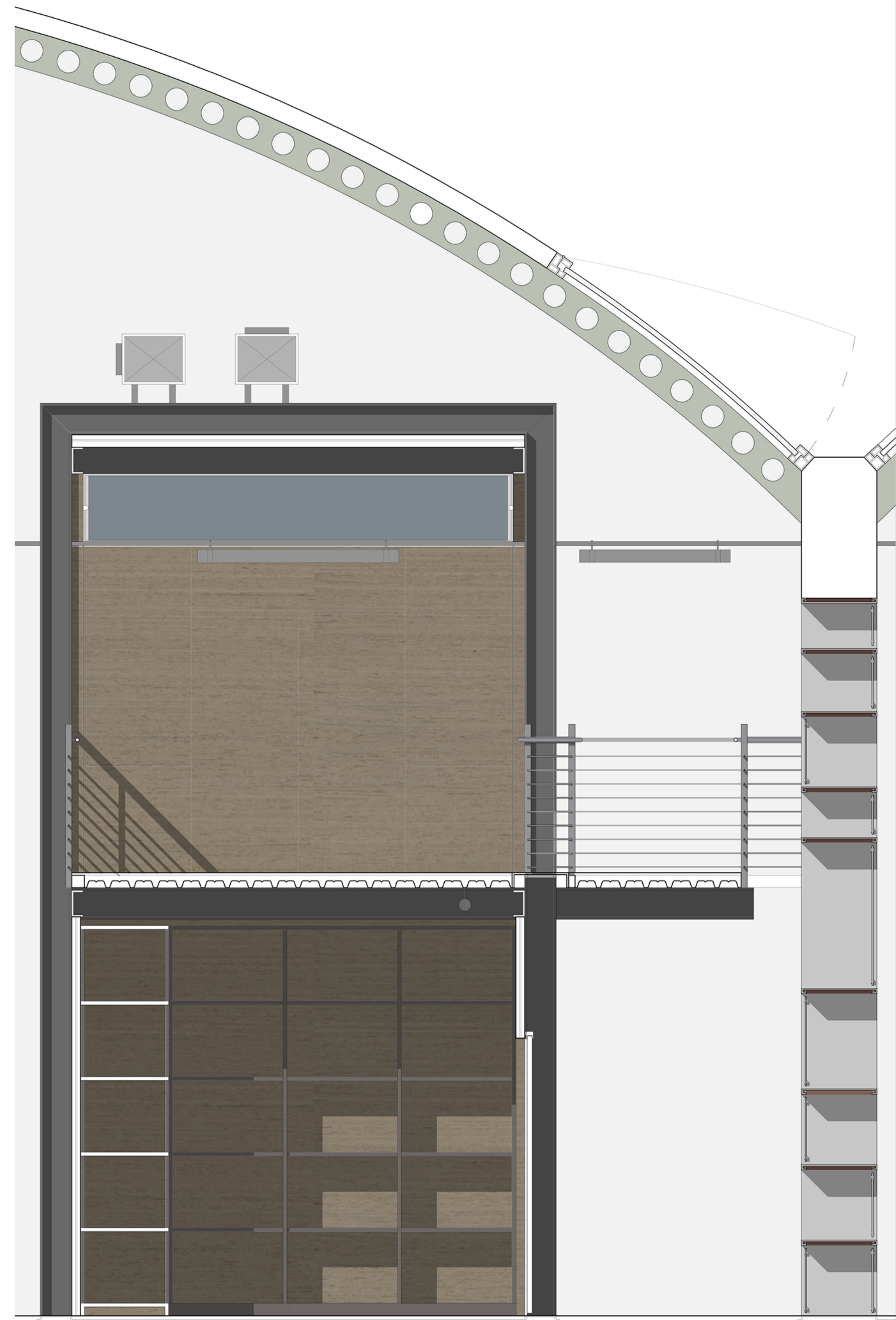
Sezione trasversale della stecca
