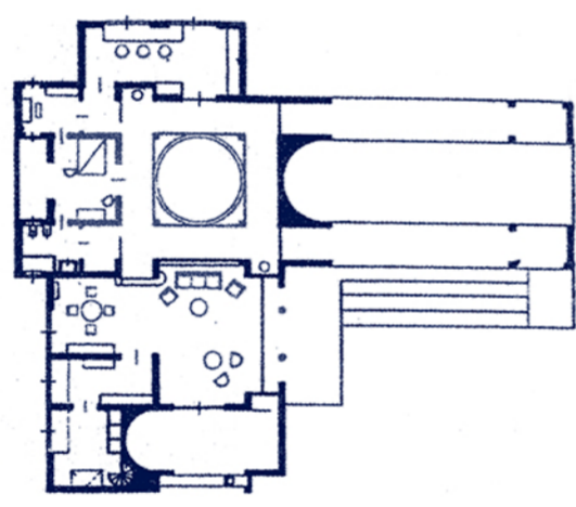
CASA SUL GOLFO _ Canino, Chiaromonte, Ceas, Sommariva _ Triennale di Milano 1933
