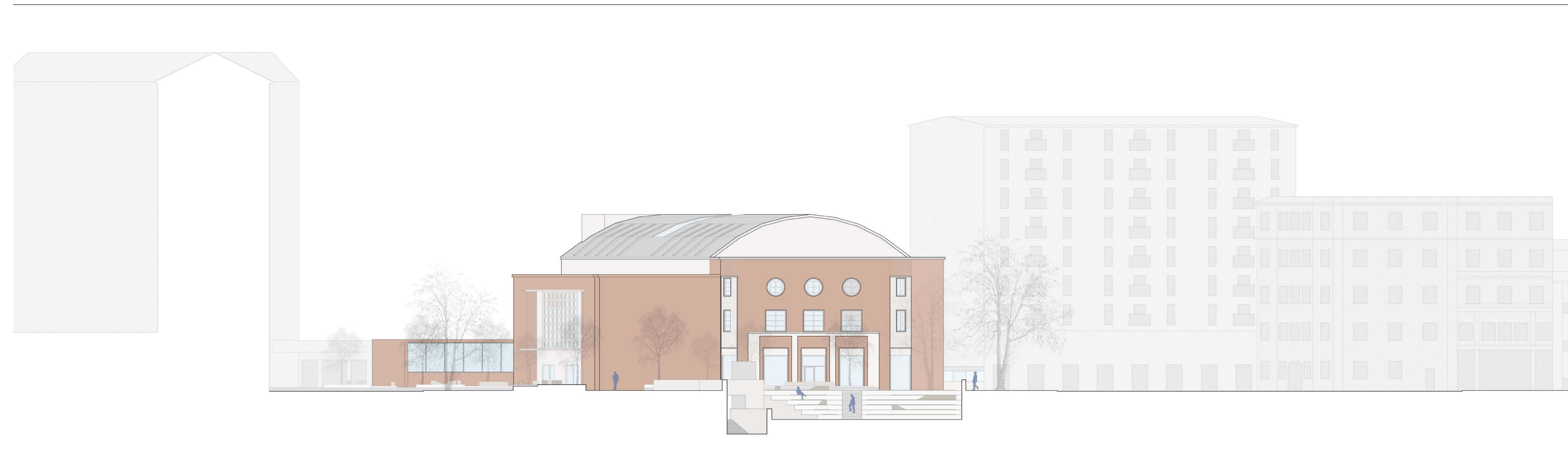
SEZIONE STRADALE B-B' _Scale 1:200
