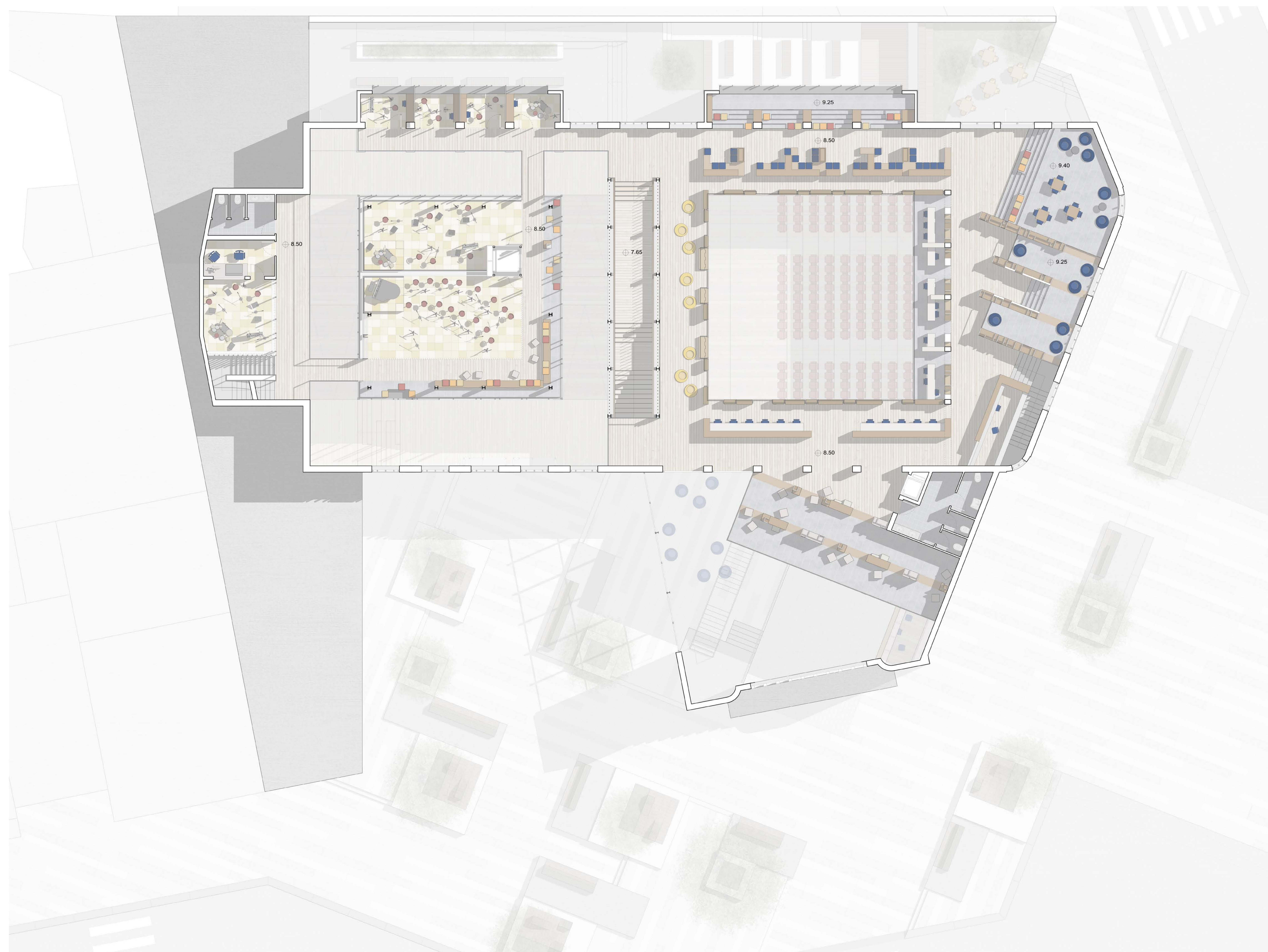
PIANTA SECONDO PIANO _Scala 1:100
