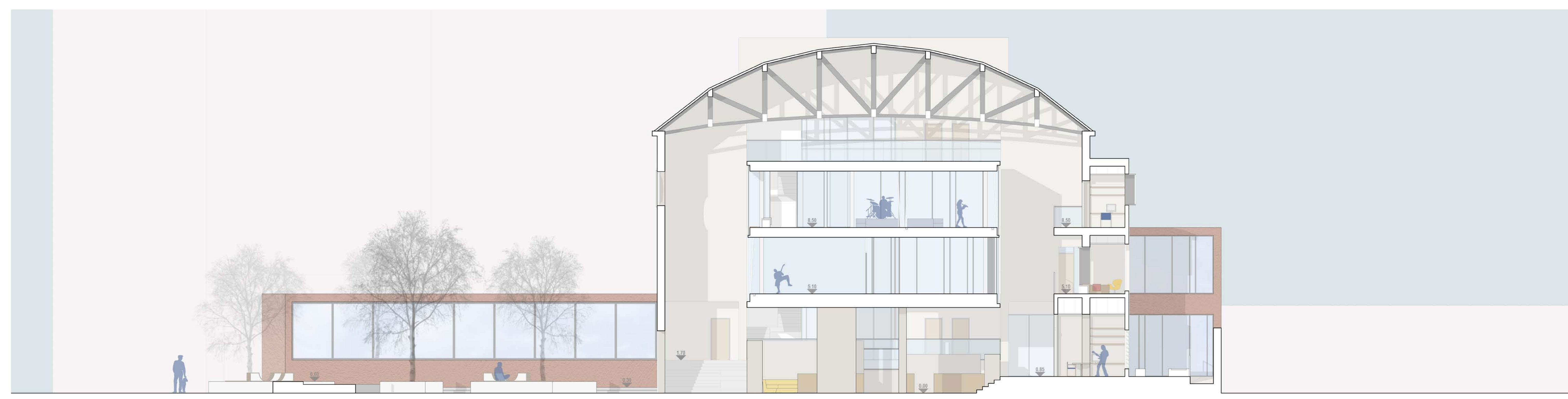
SEZIONE F-F' _Scala 1:100
