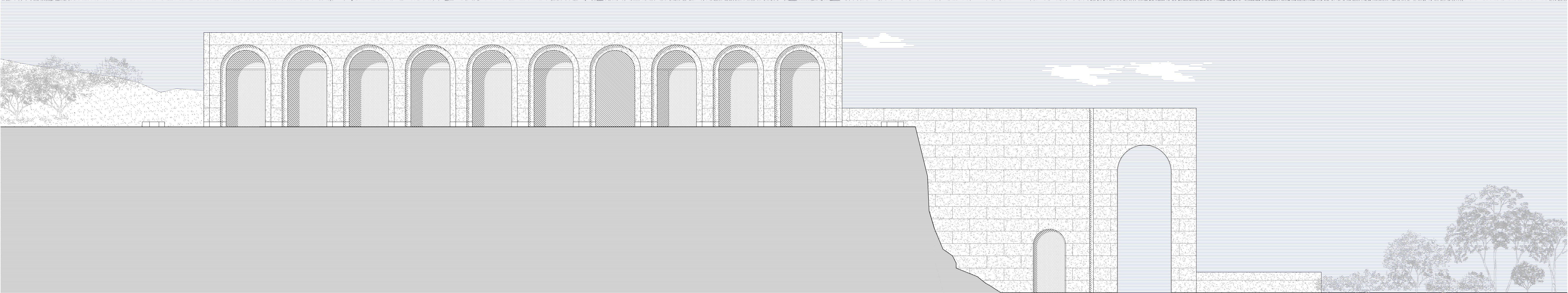
PROSPETTO OVEST ANTIQUARIUM
