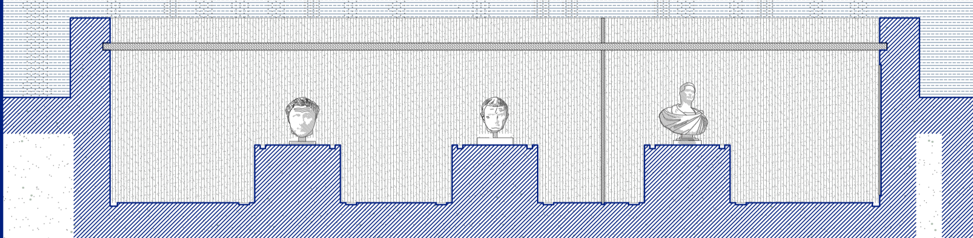
SEZIONE AA
