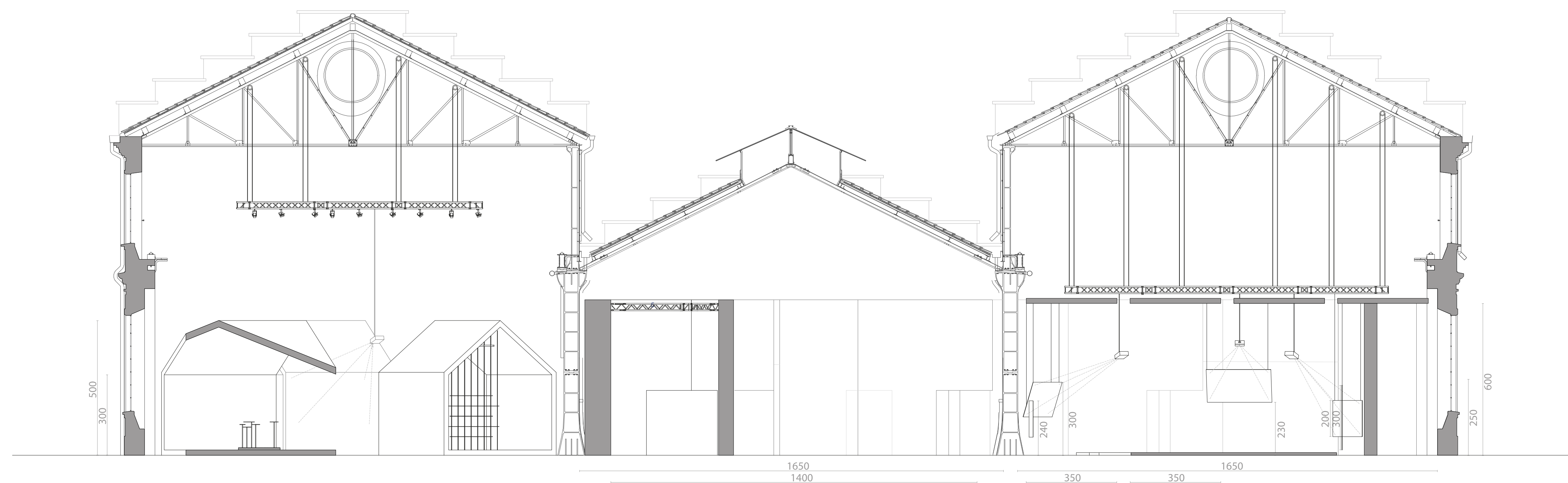
Sezione A-A' - Scala 1:100
