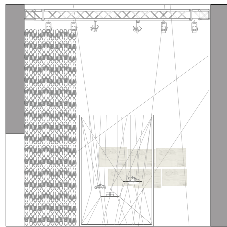
Sezione B-B'
