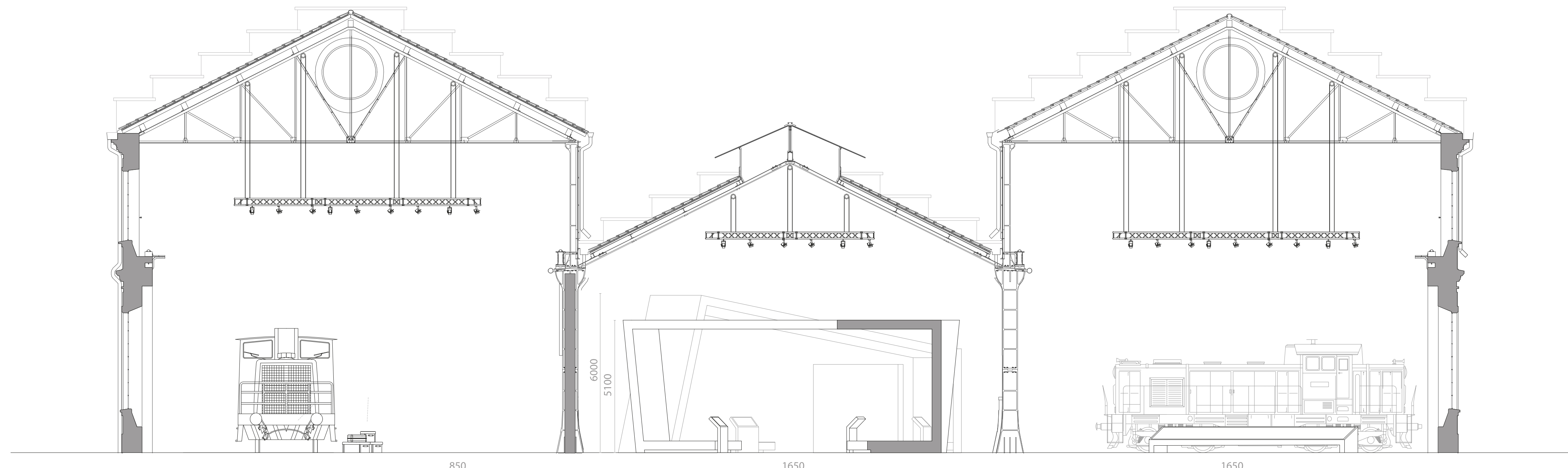
Sezione A-A' - Scala 1:100
