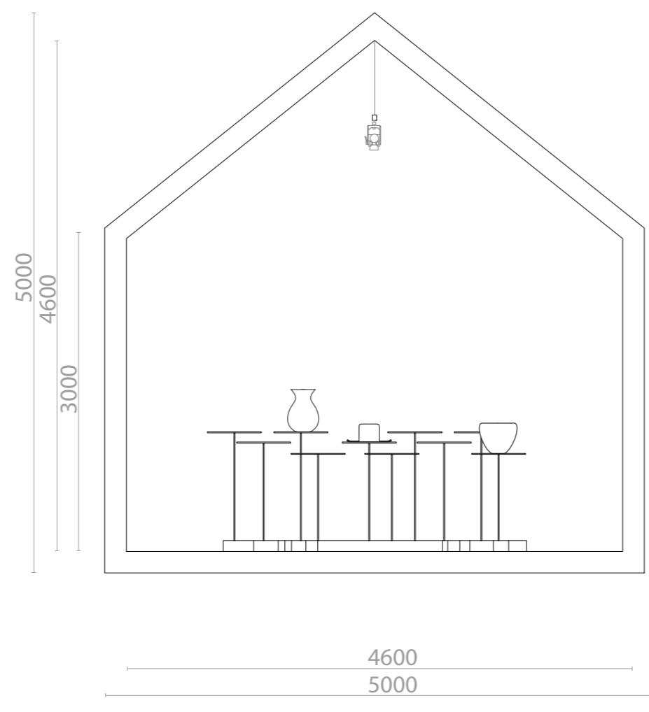
Prospetto frontale
