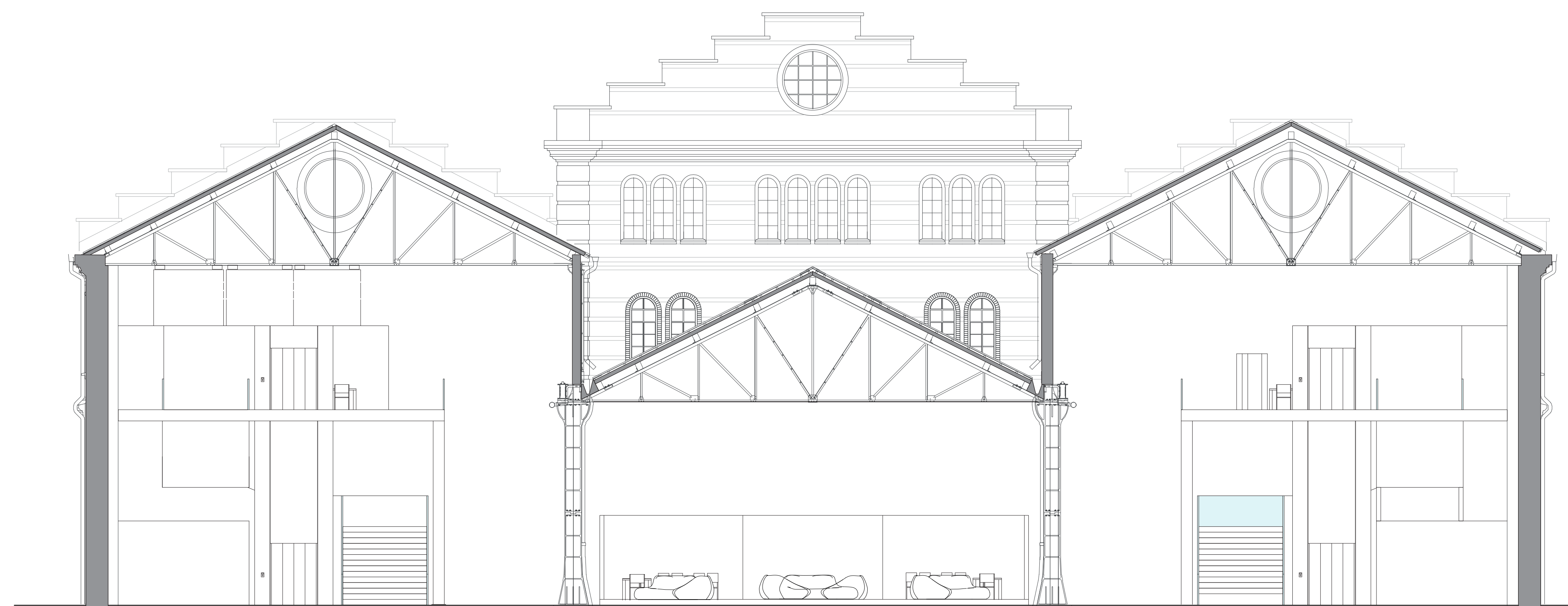
Sez. E-E' Scala 1:100
