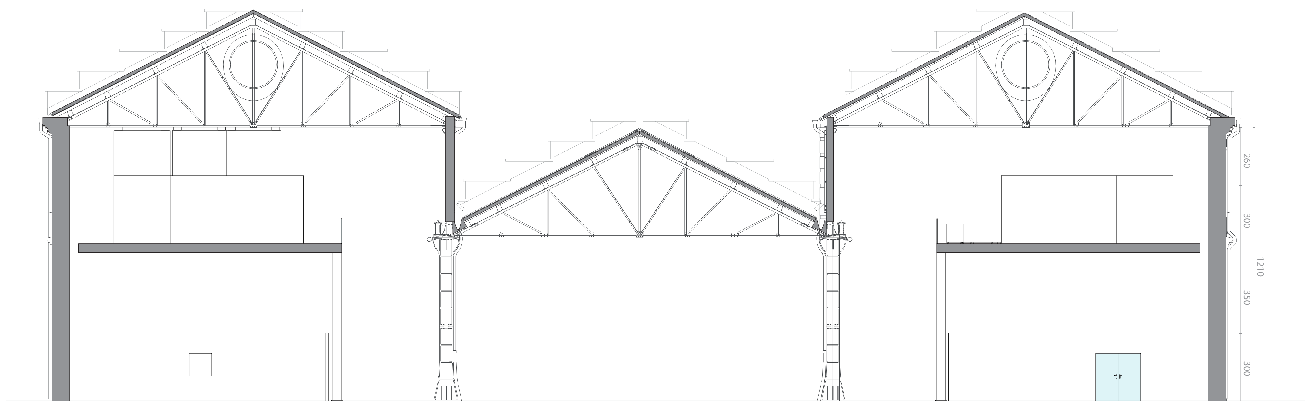
Sez. D-D' Scala 1:100 Quote in cm
