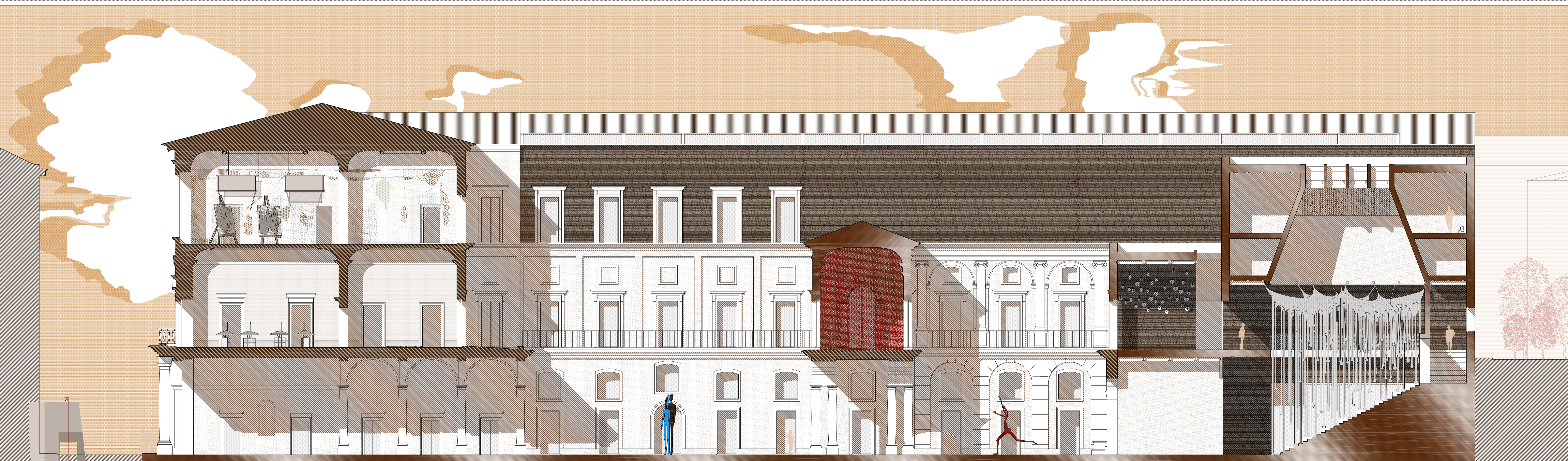
Prospetto storico Palazzo Belmonte Riso Scala 1:200
