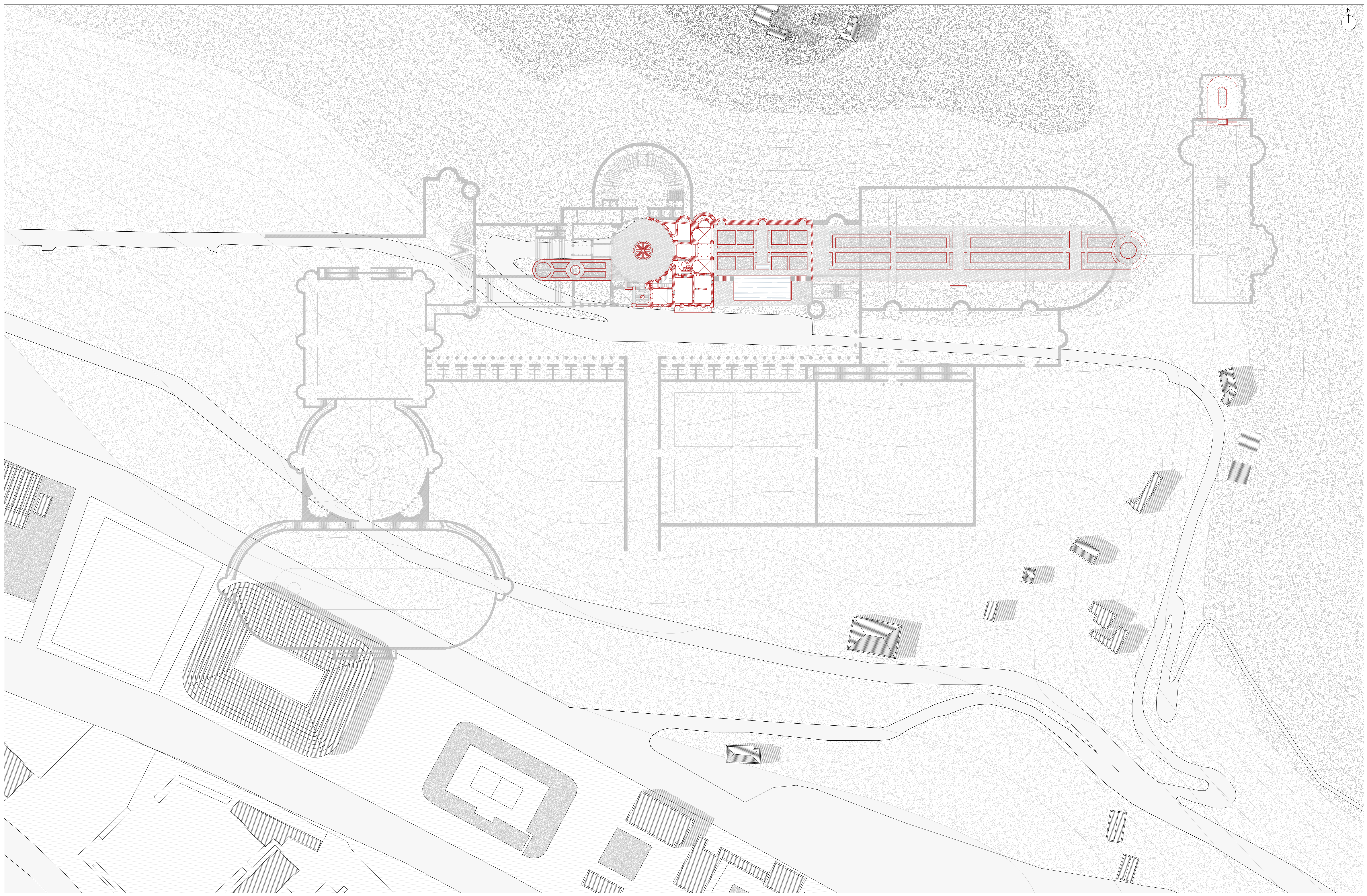
VILLA MADAMA SOVRAPPOSIZIONE STATO ATTUALE - PROGETTO ORIGINARIO
