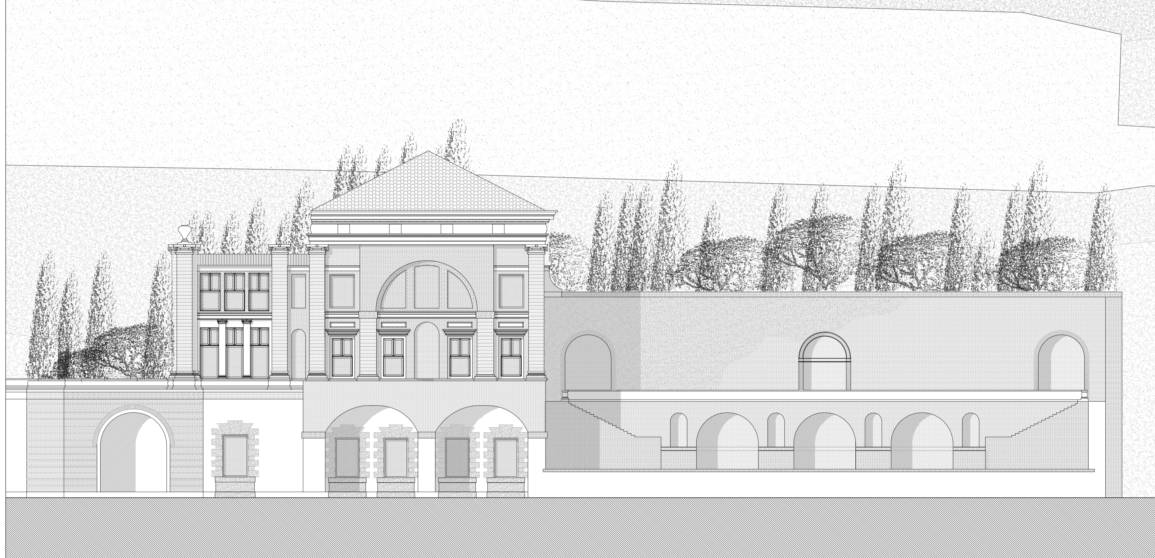
VILLA MADAMA RIDISEGNO DELL'ESISTENTE SCALA 1:200
