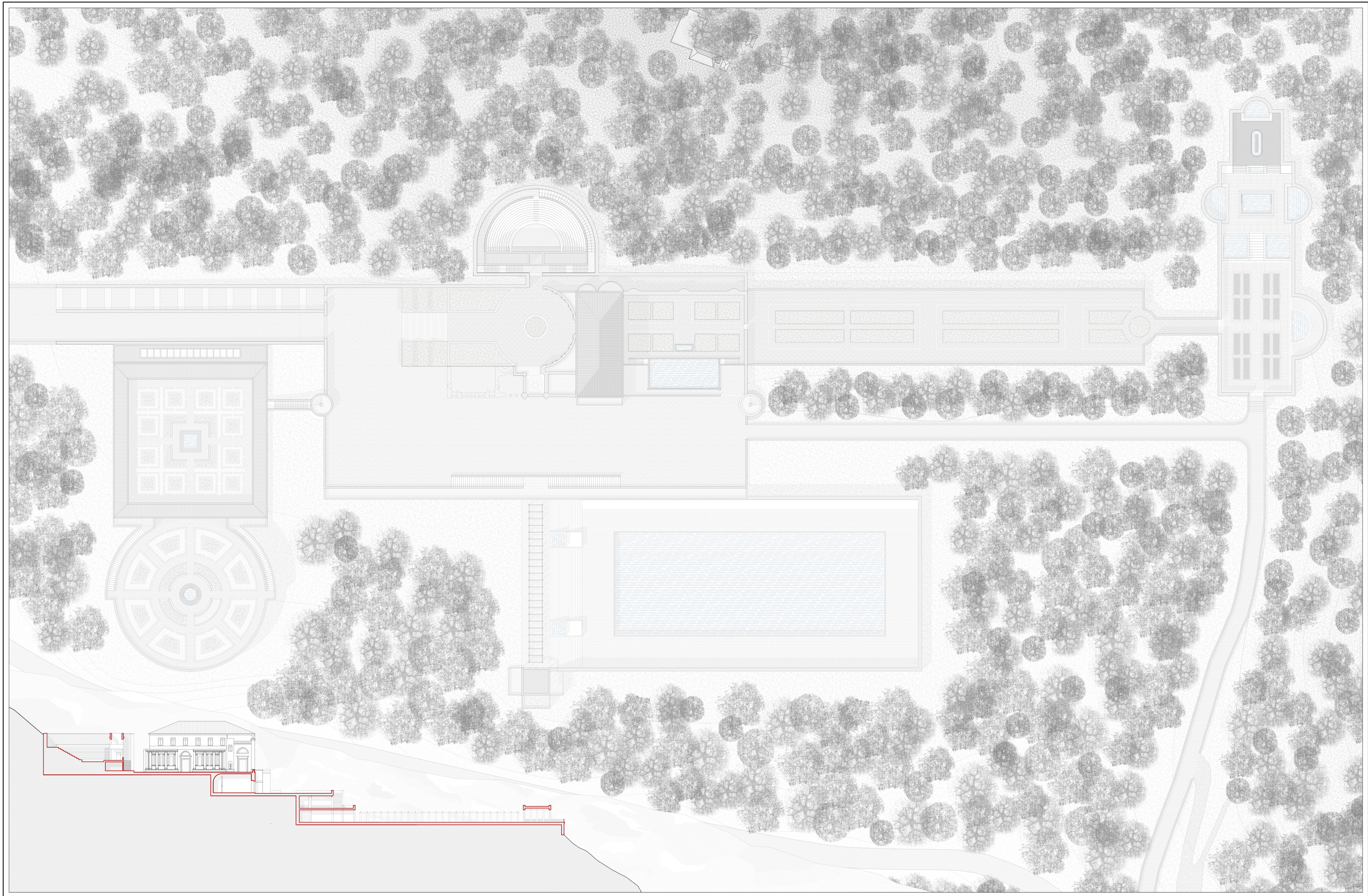
VILLA MADAMA PLANIVOLUMETRICO E SEZIONE
