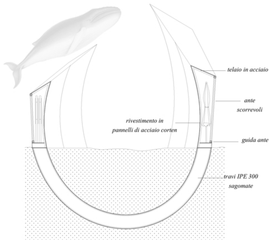
sezione assonometrica scala 1:50
