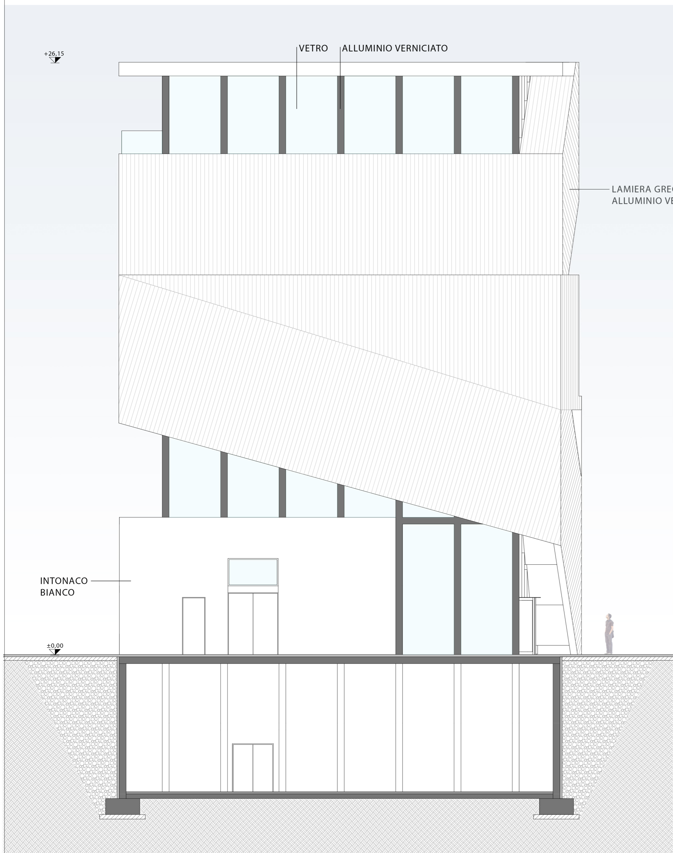
PROSPETTO EST 1:100
