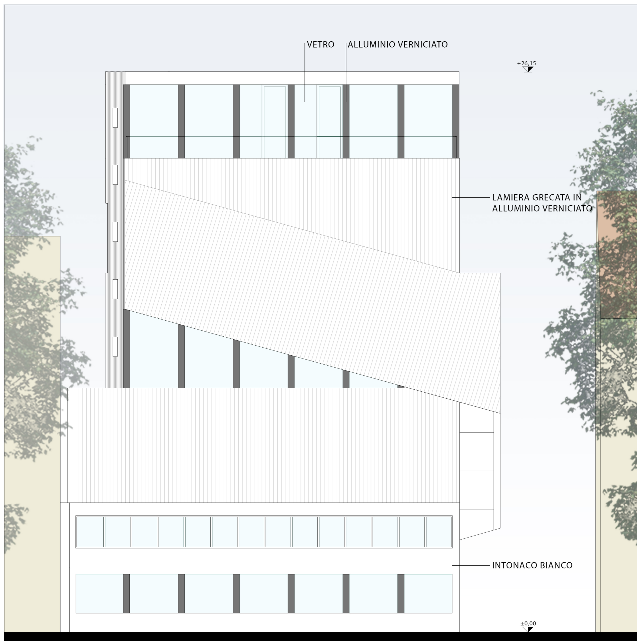
PROSPETTO SUD 1:100
