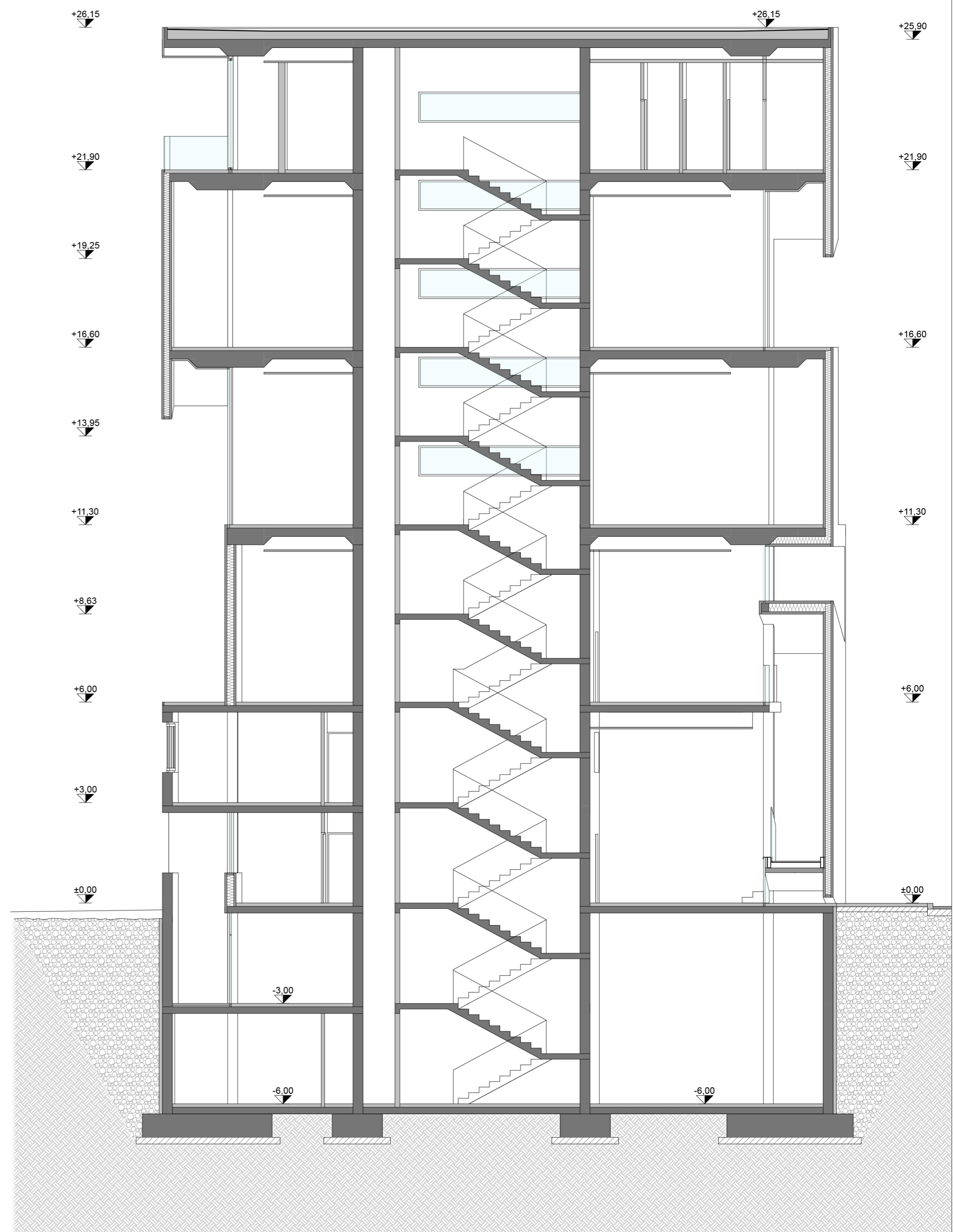
SEZIONE 3-3' 1:100
