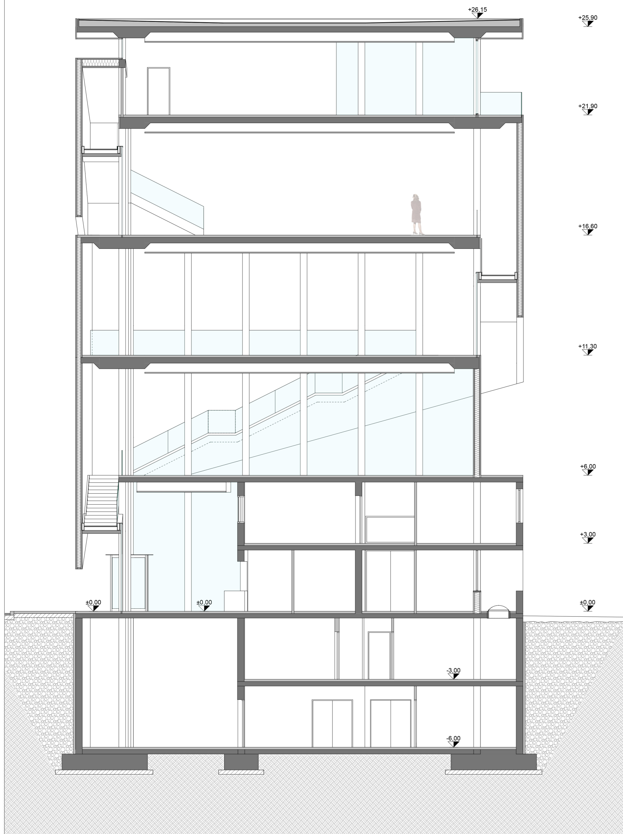
SEZIONE 2-2' 1:100
