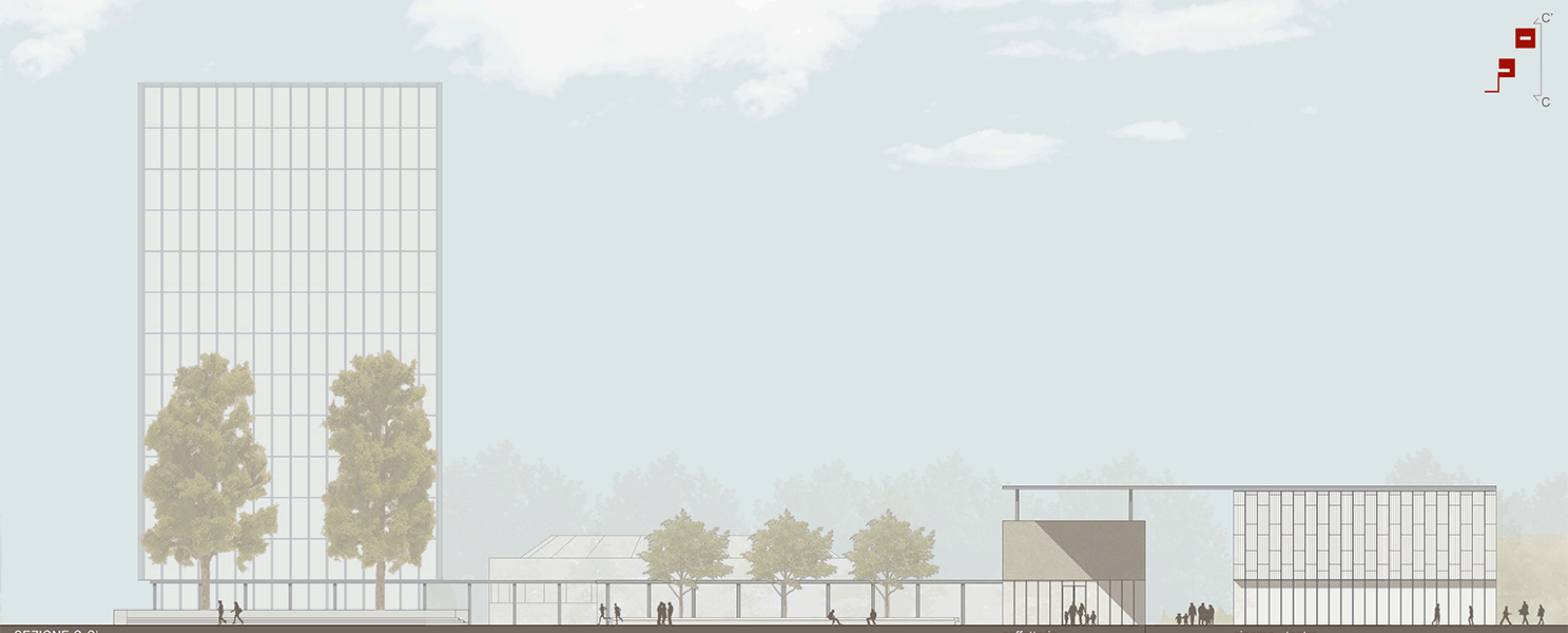
SEZIONE C-C'
