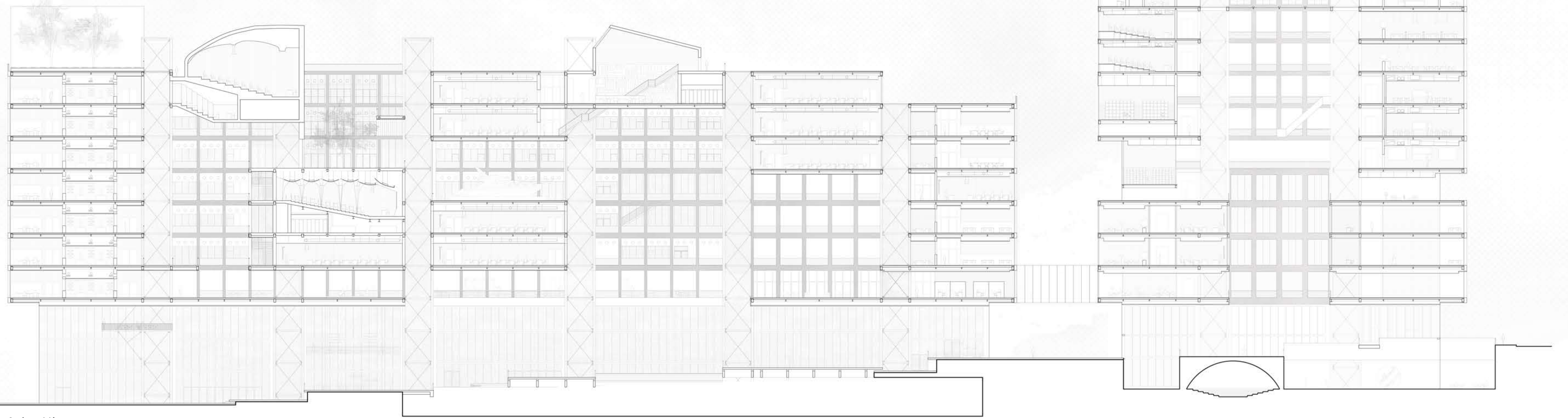
Sezione AA'
