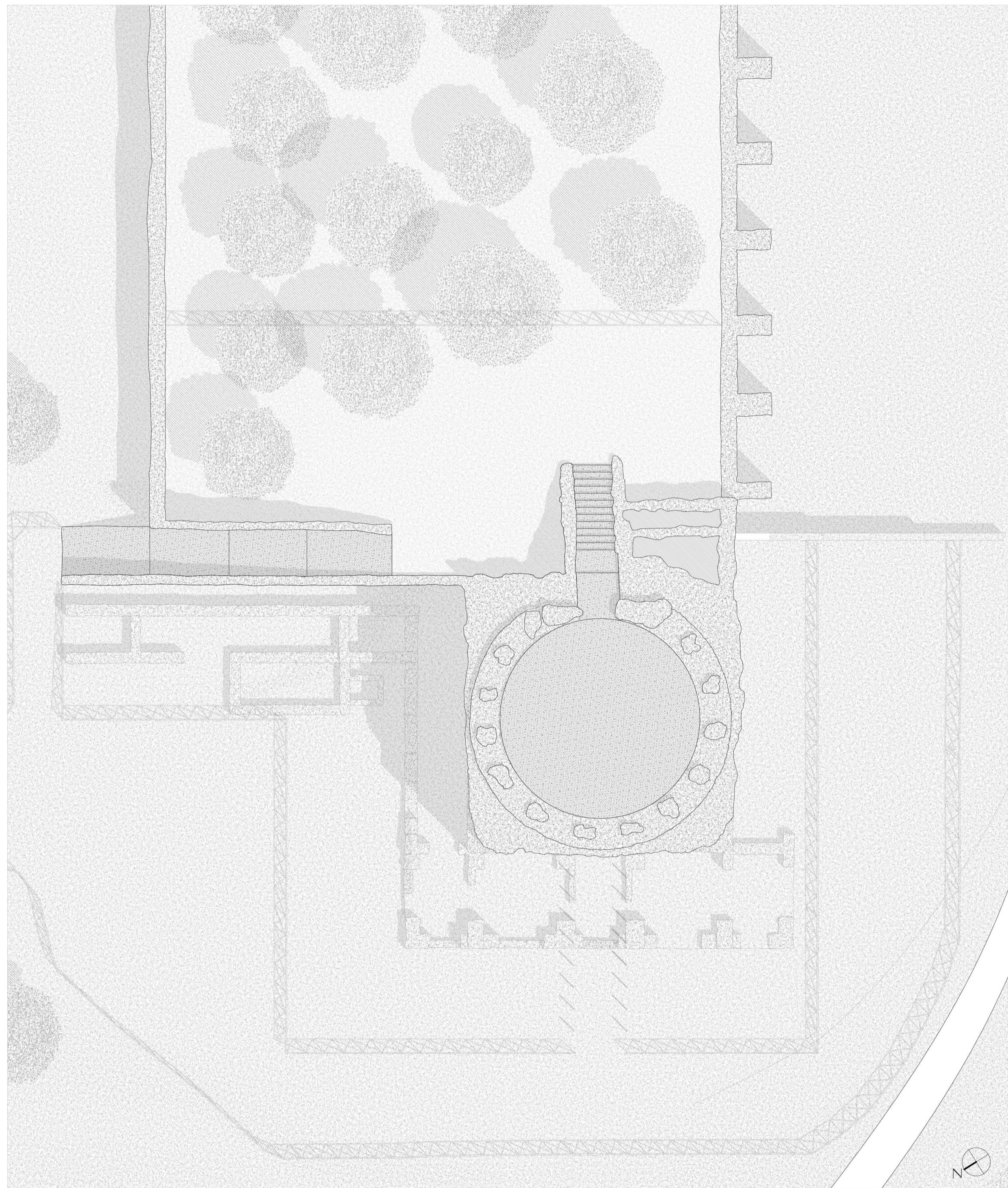
PIANTA STATO DI FATTO SCALA 1:200
