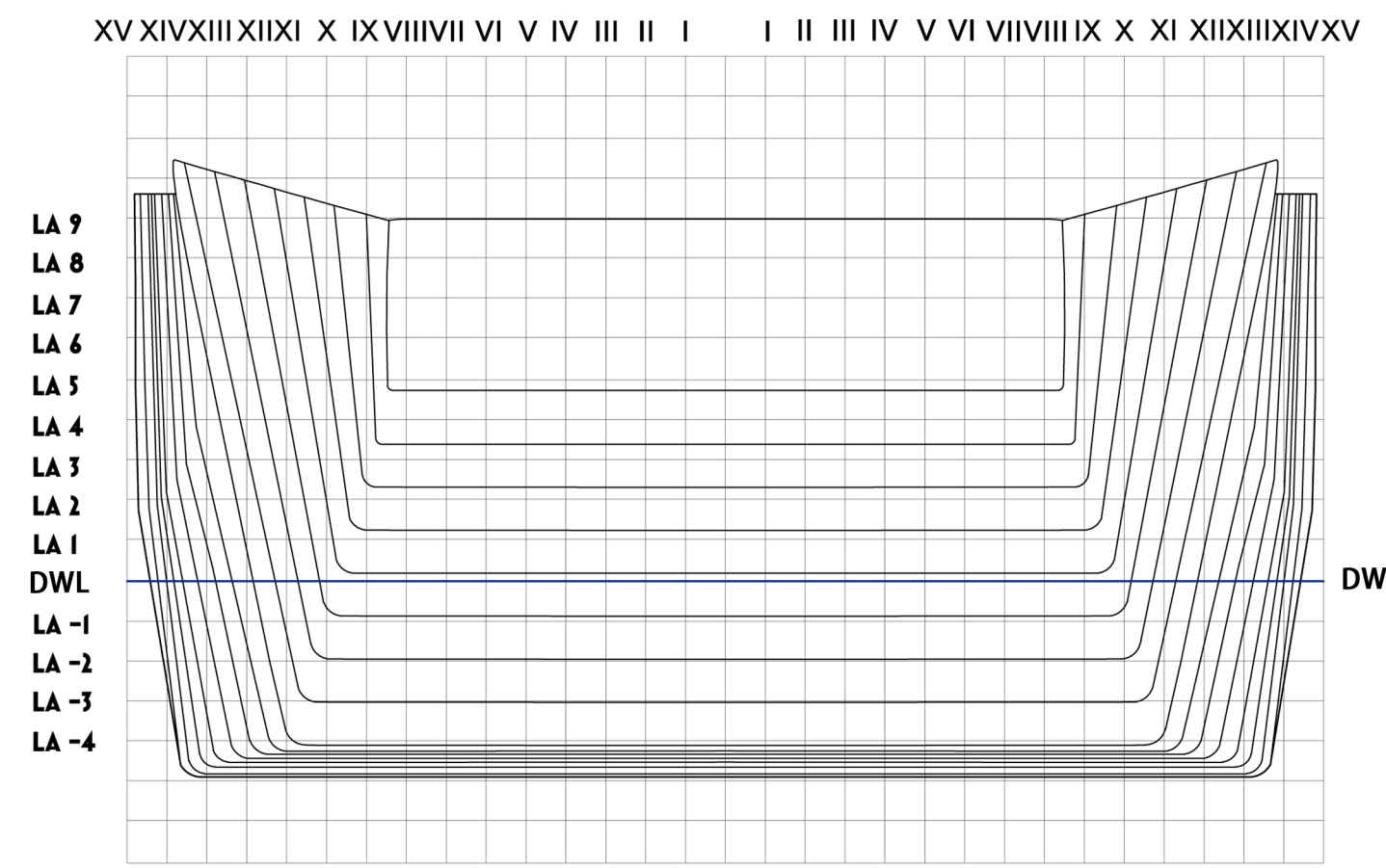
PIANO DELLE ORDINATE _ PRUA
