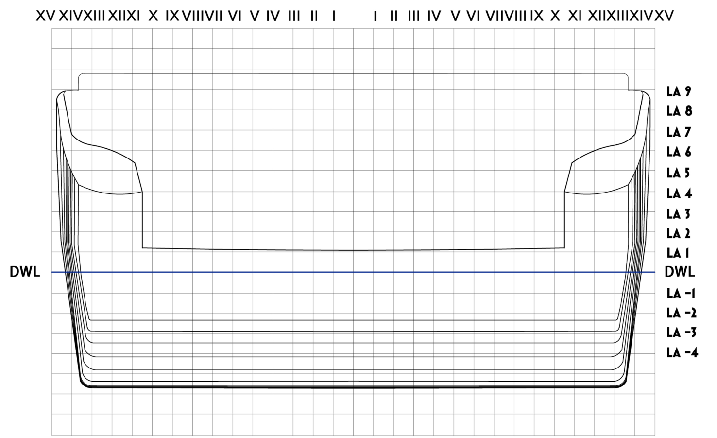
PIANO DELLE ORDINATE _ POPPA
