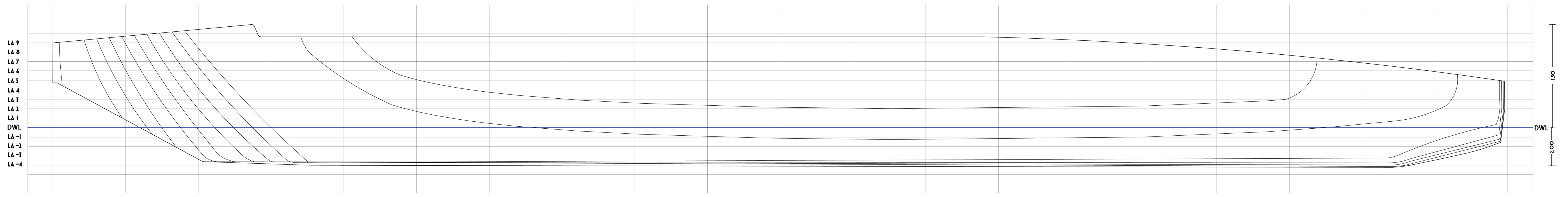
PIANO DEI PROFILI _ PROFILO LATERALE
