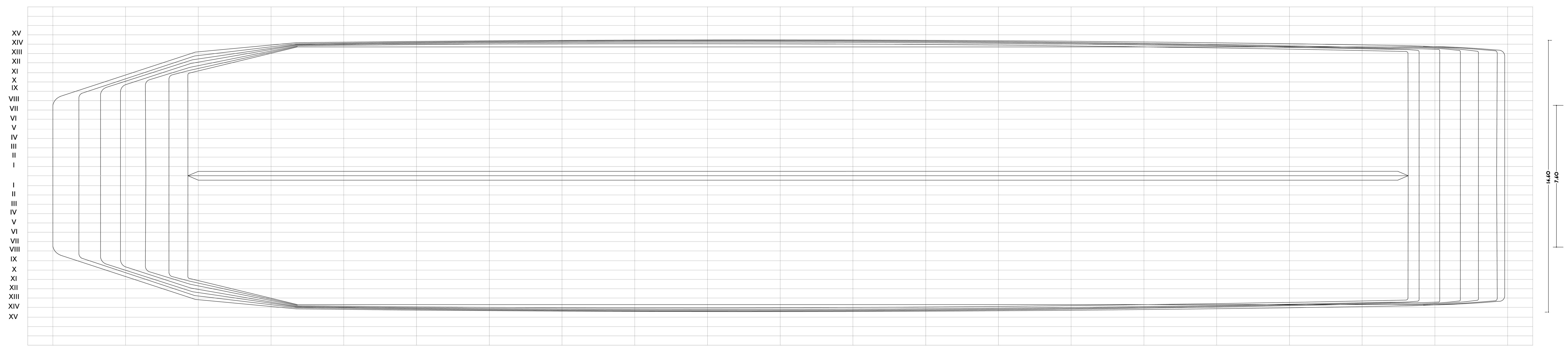
PIANO DELLE LINEE D' ACQUA _ PIANTA
