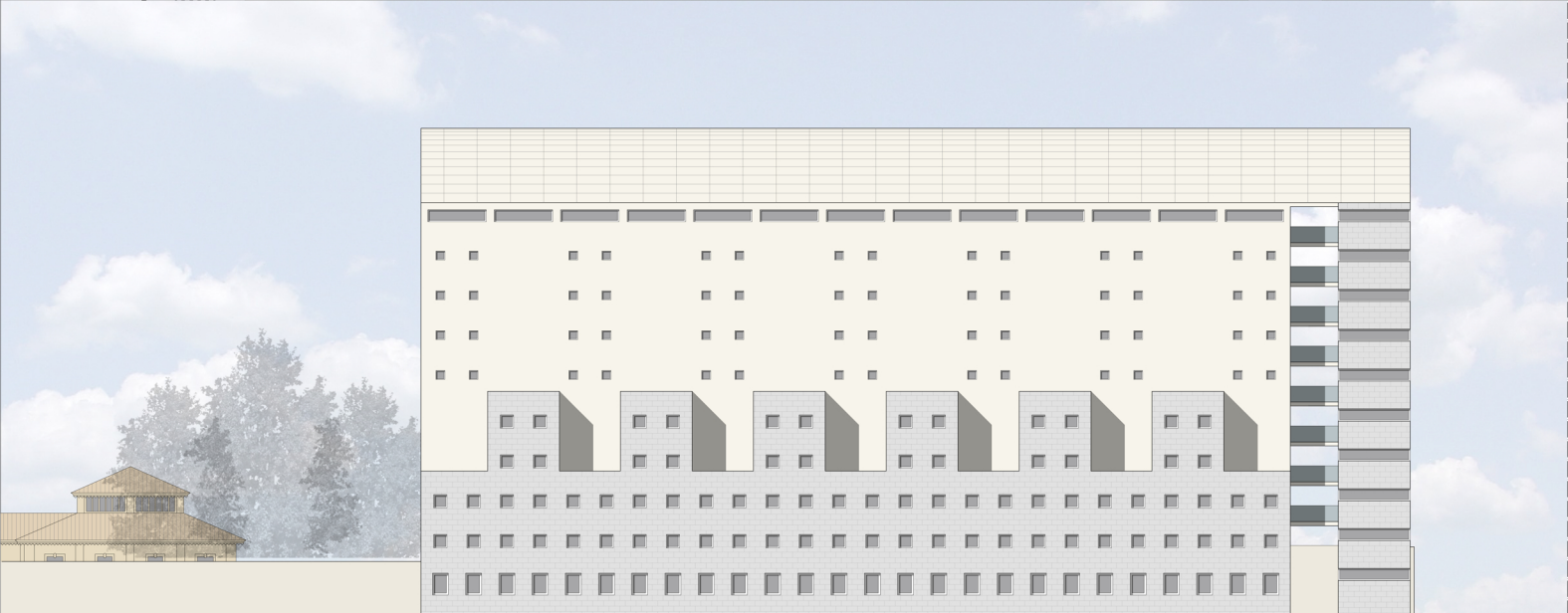
Prospetto esterno
