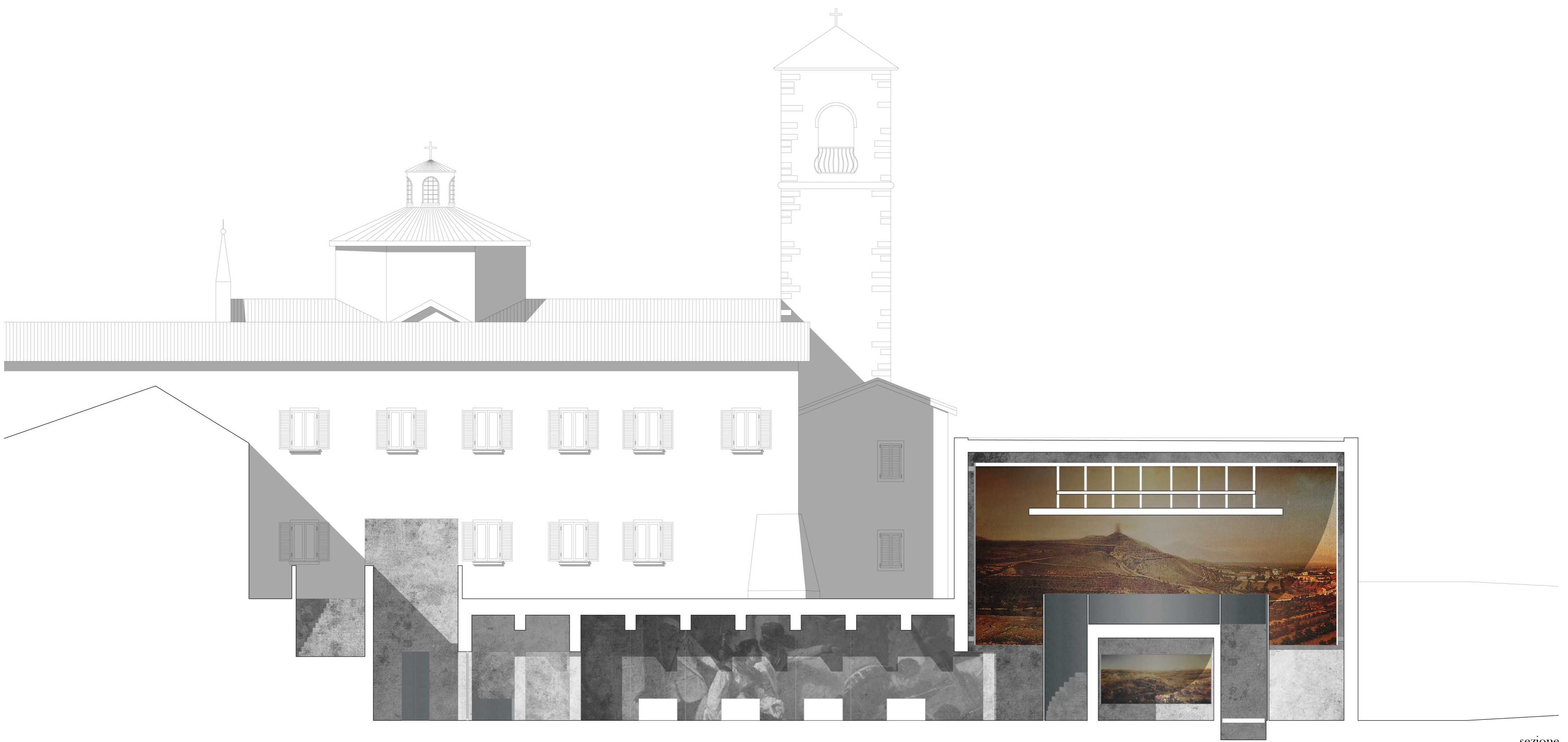
sezione 1:100
