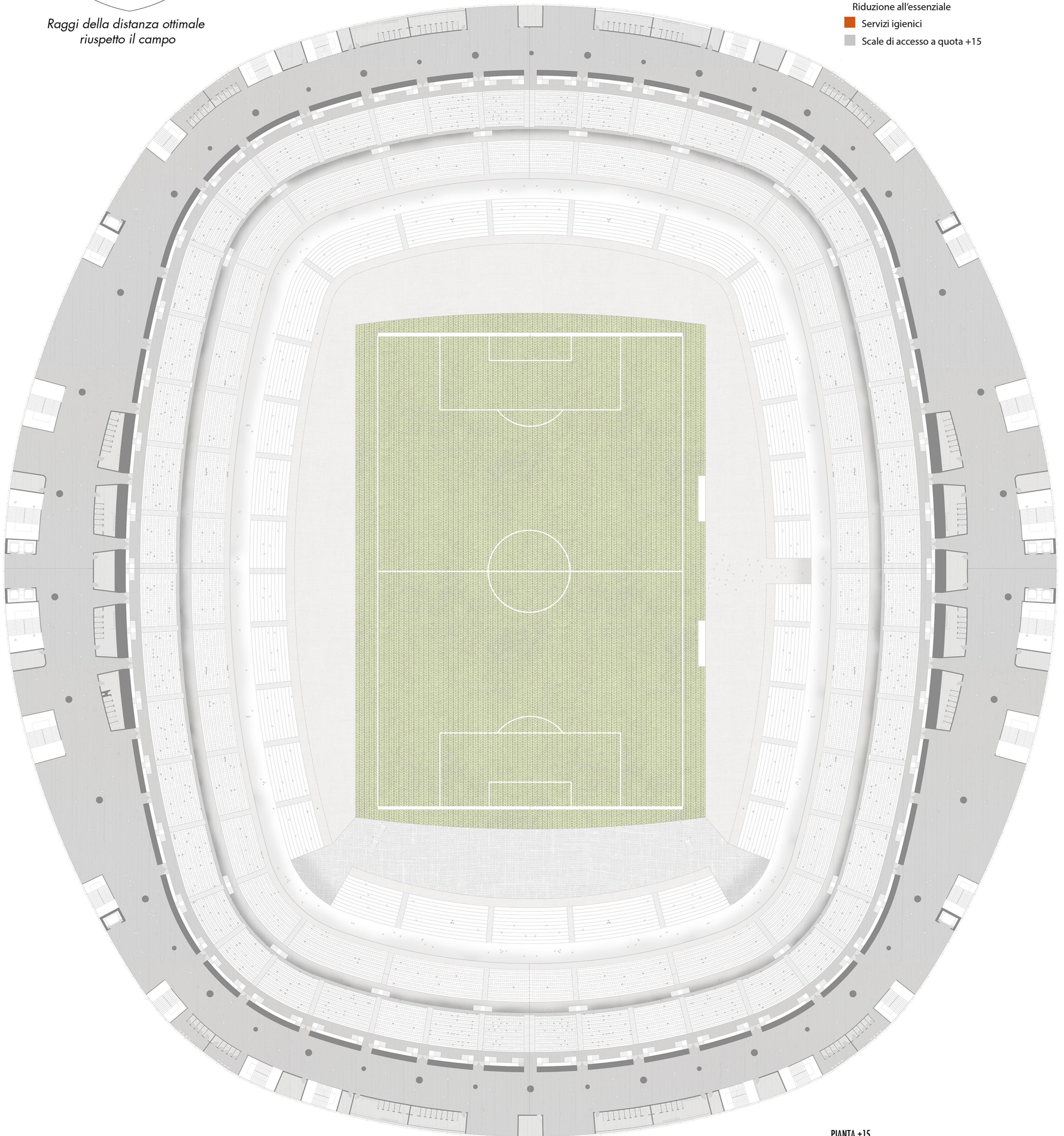
PIANTA +15 SCALA 500
