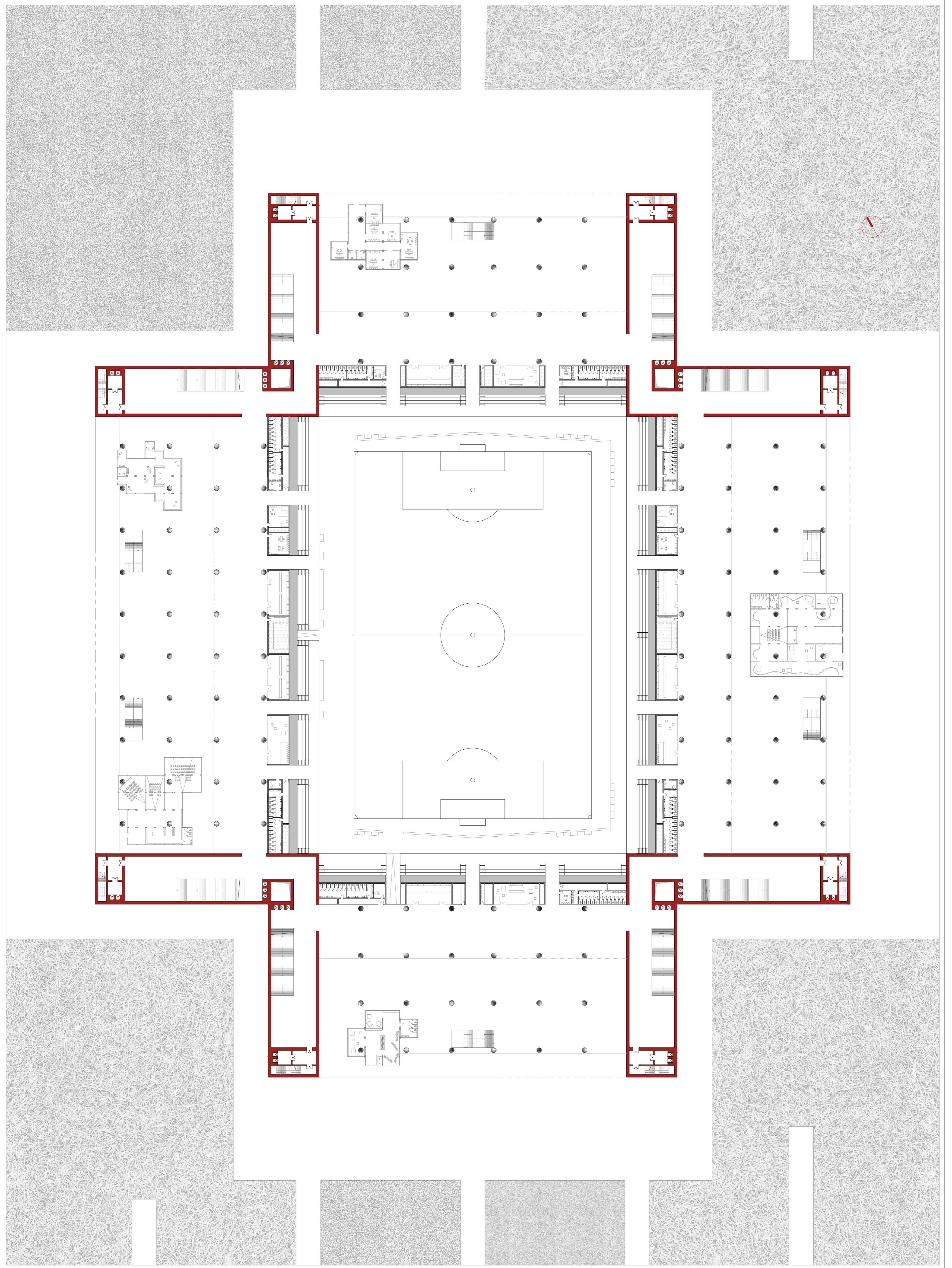
PIANTA LIVELLO ZERO + 0.00 m Scala 1:500
