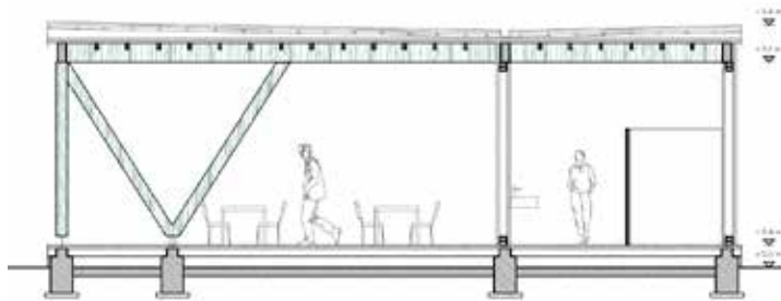
sezione trasversale
