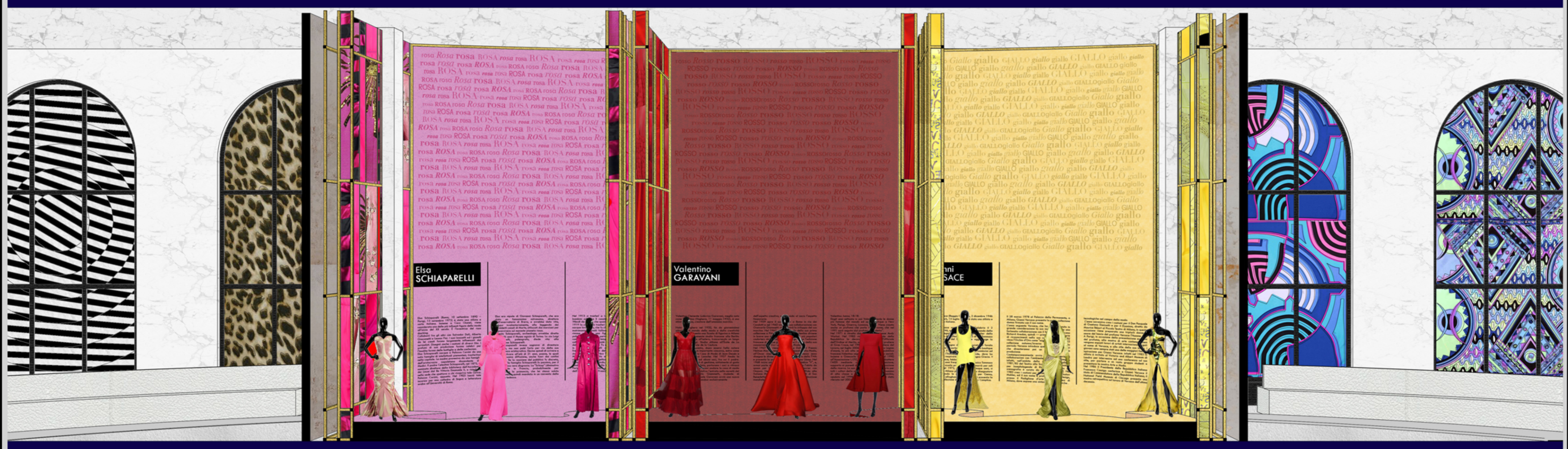
sezione AA' 1: 50
