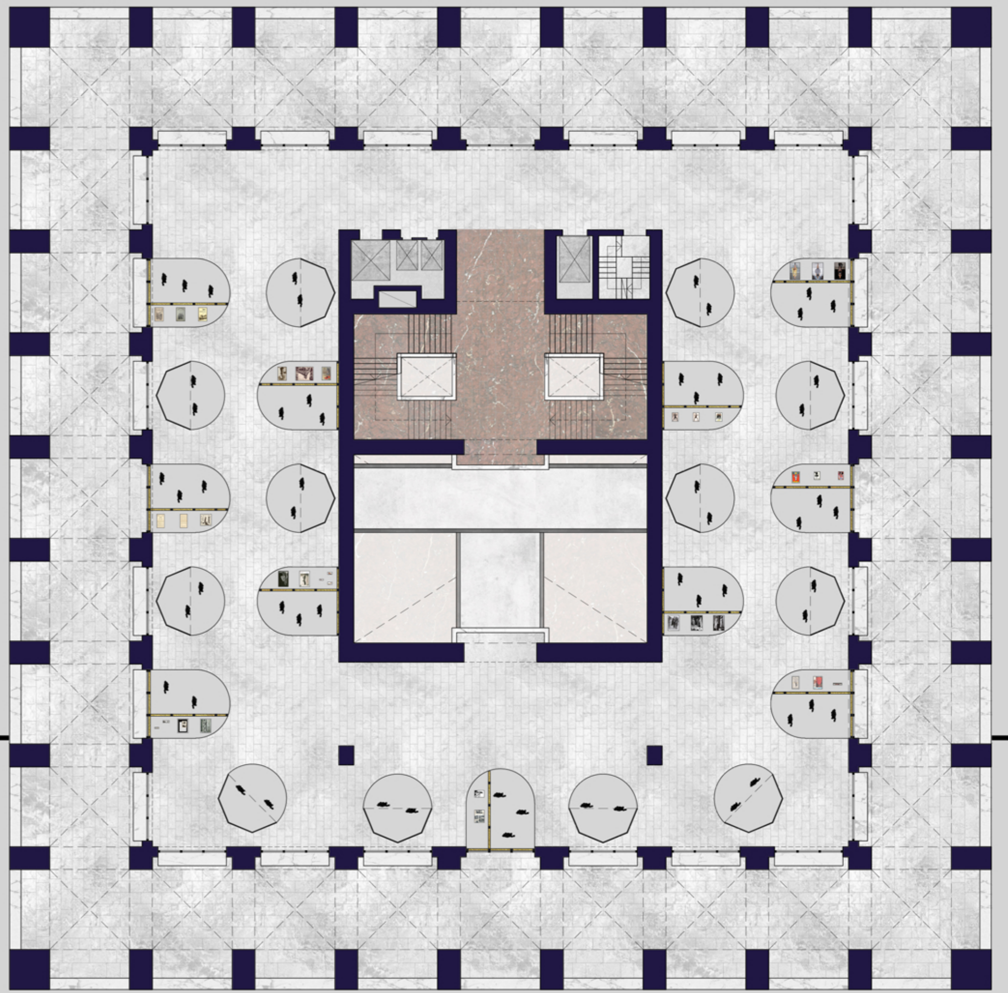
◆ pianta p.IV 1:200
